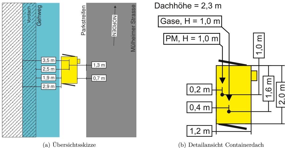
Abbildung 3: Schematische Darstellung - Oberhausen Mülheimer Straße
