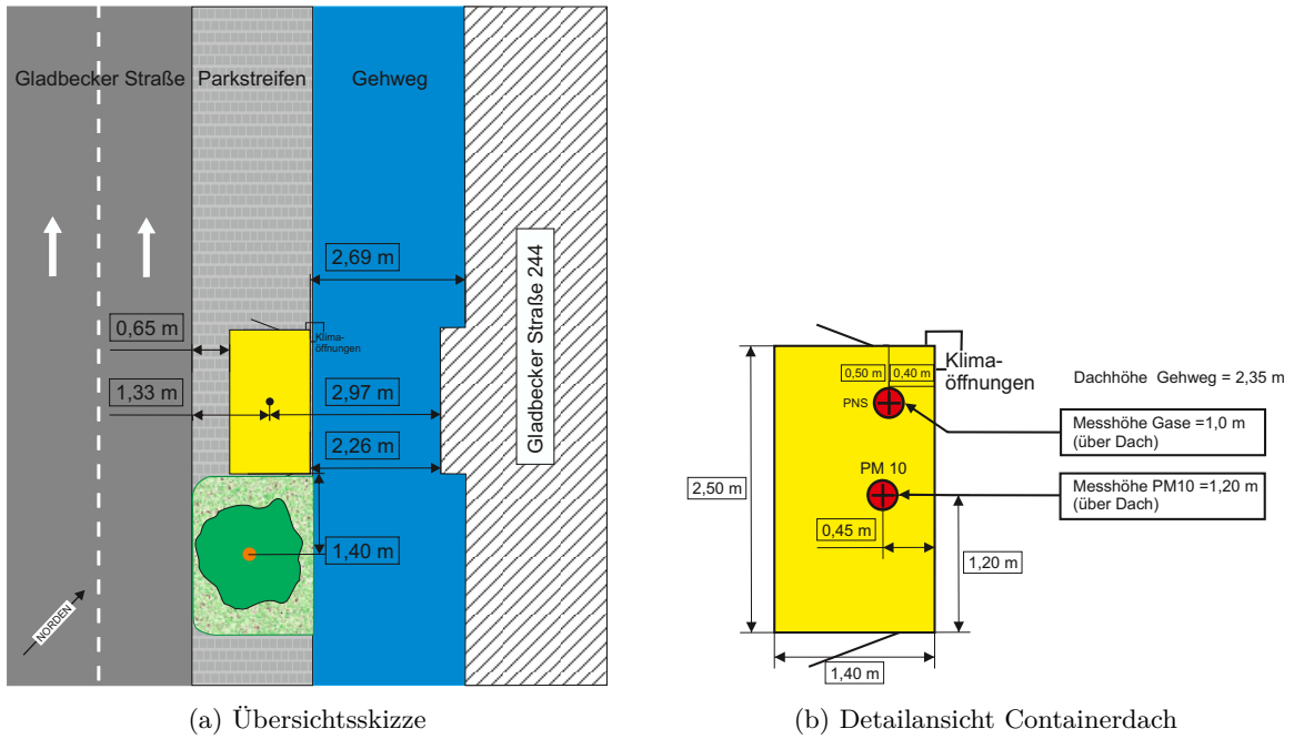
Abbildung 3: Schematische Darstellung - Essen Gladbecker Straße
