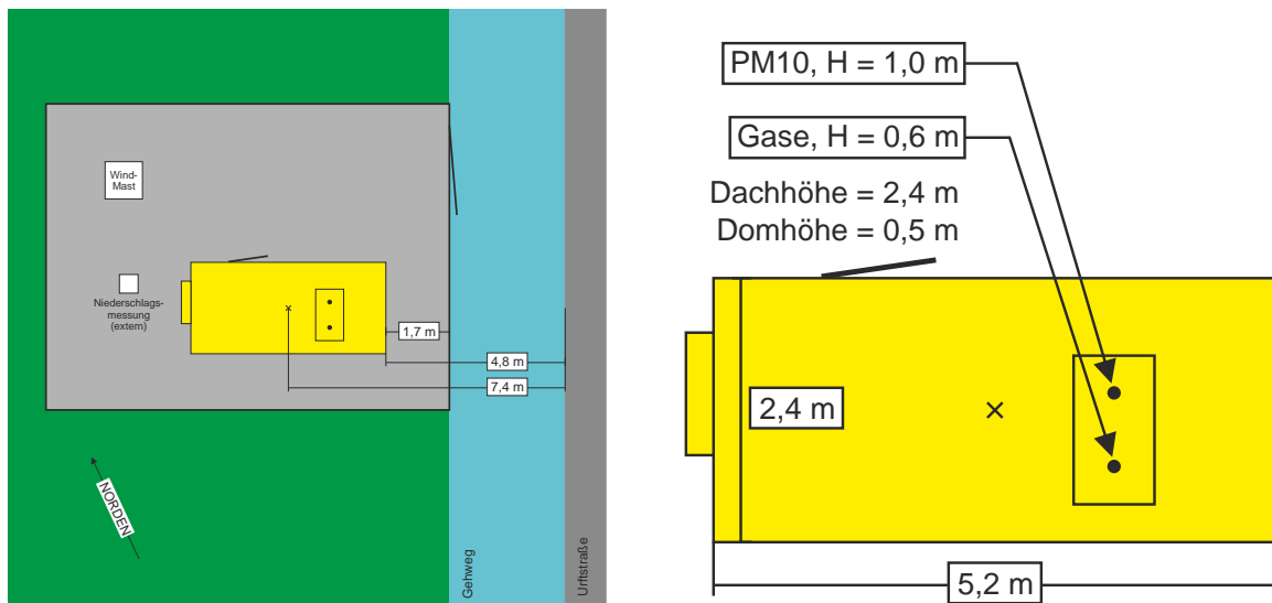
(a) Übersichtsskizze
