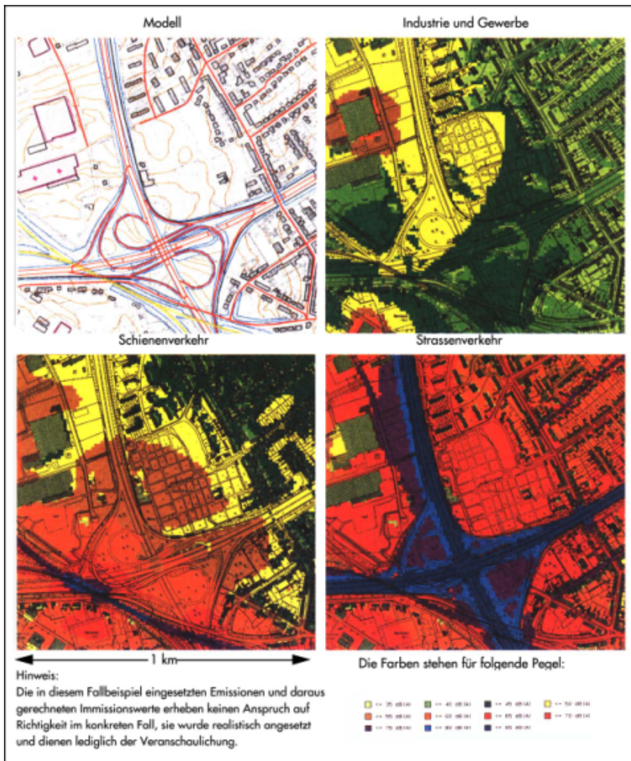
Bild 2: Fallstudie einer Gelande, Hindernis- und Quellenmodellierung mit daraus gerechneten Ergebnissen fur die Quellengruppe Strae, Schiene und Industrie & Gewerbe.
