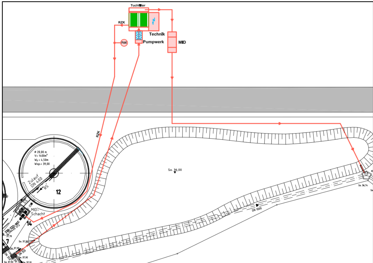
Abbildung 9.5: Mögliche Ausführungsform der Variante 1.3
