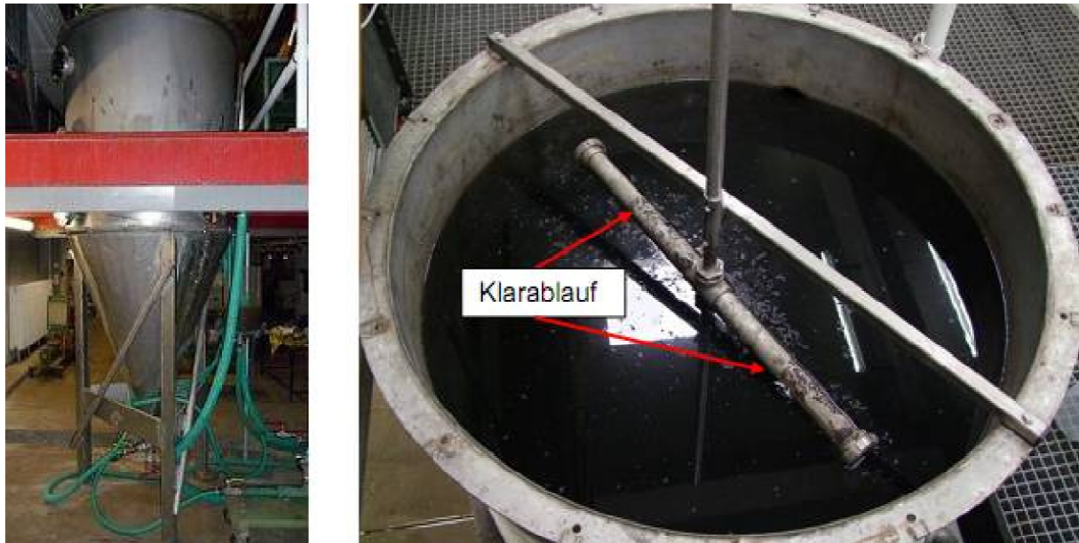
Abbildung 5.21: Sedimentationsreaktor (Pinnekamp, 2012)
