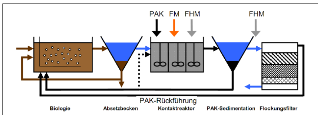
Abbildung 5.19: AFSF-Verfahrensschema (Pinnekamp, 2012)
