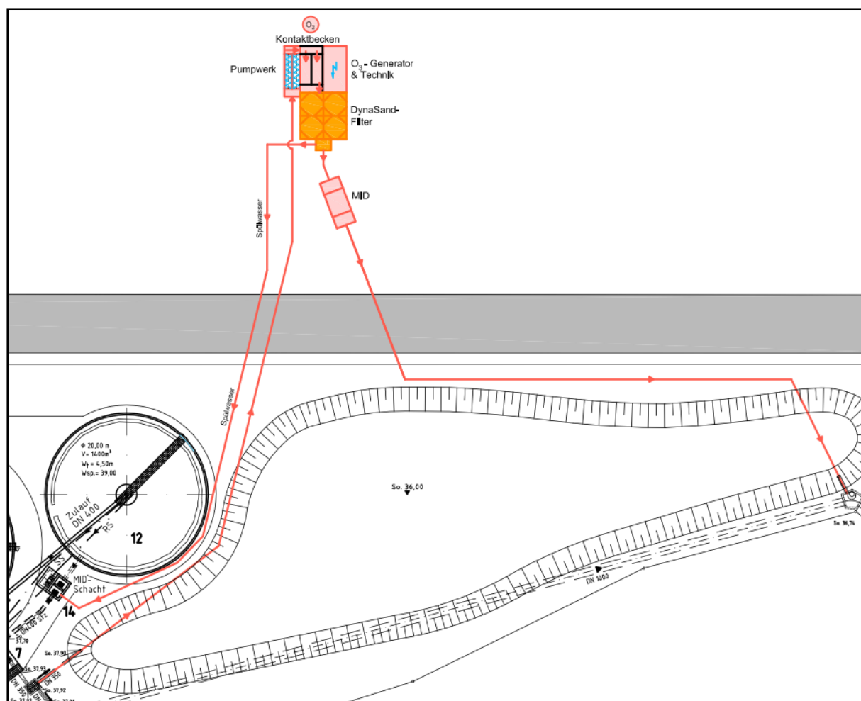
Abbildung 9.9: Mögliche Ausführungsform der Variante 3 auf der Kläranlage Saerbeck
