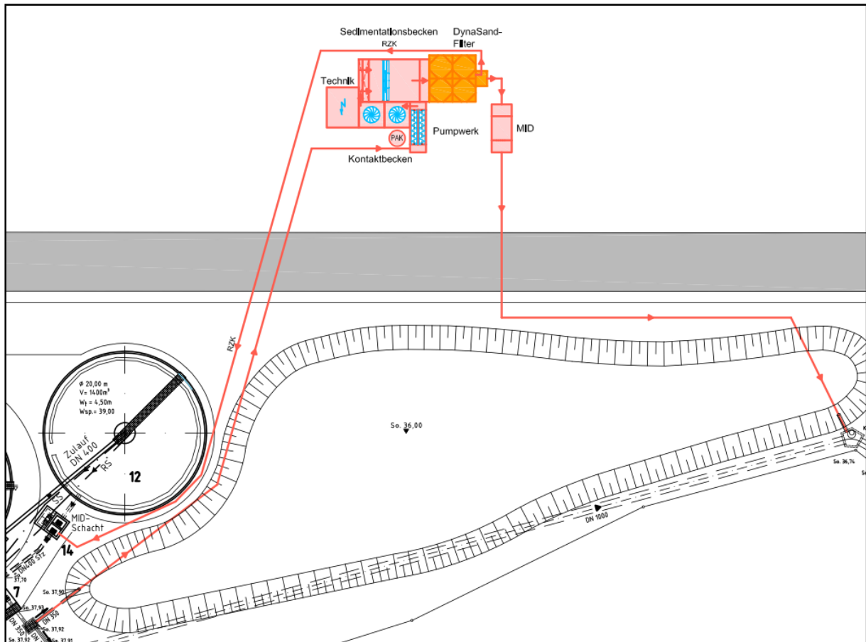
Abbildung 9.1: Mögliche Ausführungsform der Variante 1.1
