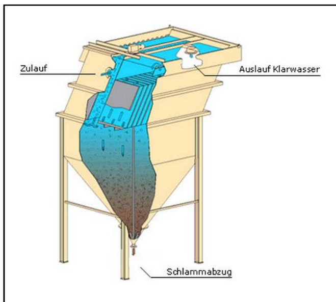
Abbildung 5.22: Funktionsprinzip des Lamellenabscheiders (Leiblein, 2013)
