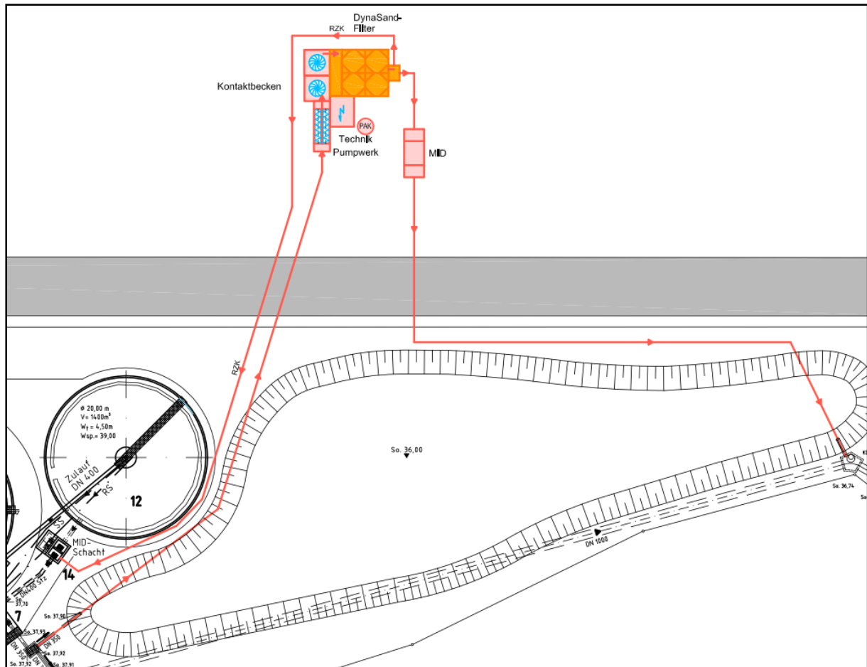
Abbildung 9.3: Mögliche Ausführungsform der Variante 1.2
