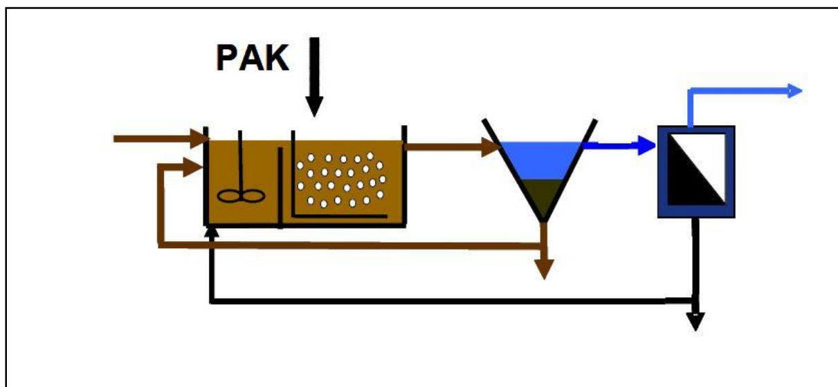
Abbildung 5.13: Vereinfachte Darstellung der Direktdosierung von PAK in die Belebungsbecken (verändert und ergänzt nach Zwickenpflug et al., 2010)
