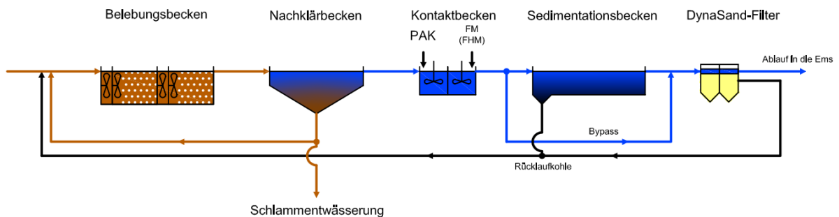
Abbildung 9.2: Fließschema zur Variante 1.1
