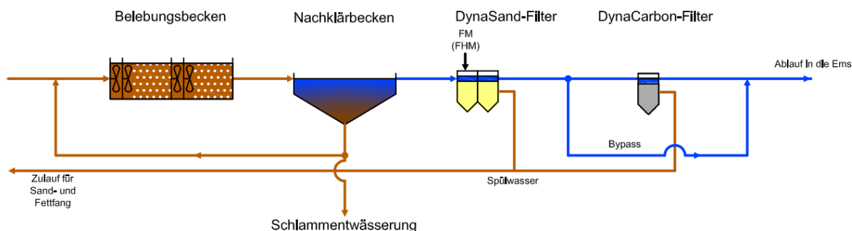
Abbildung 9.8: Fließschema der Variante 2
