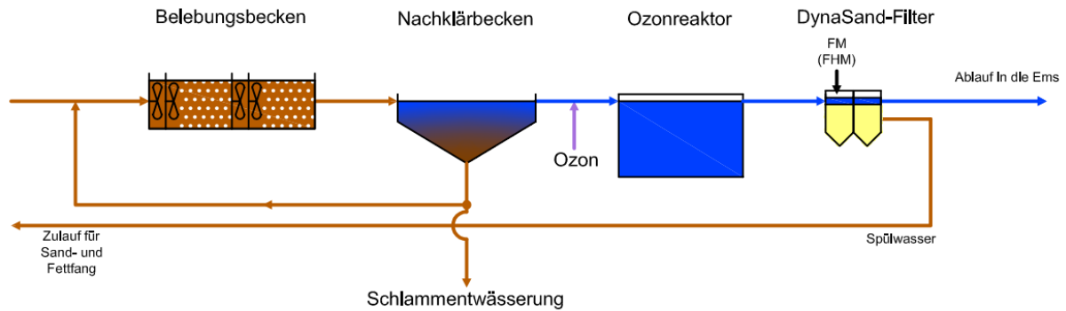
Abbildung 9.10: Fließschema der Variante 3
