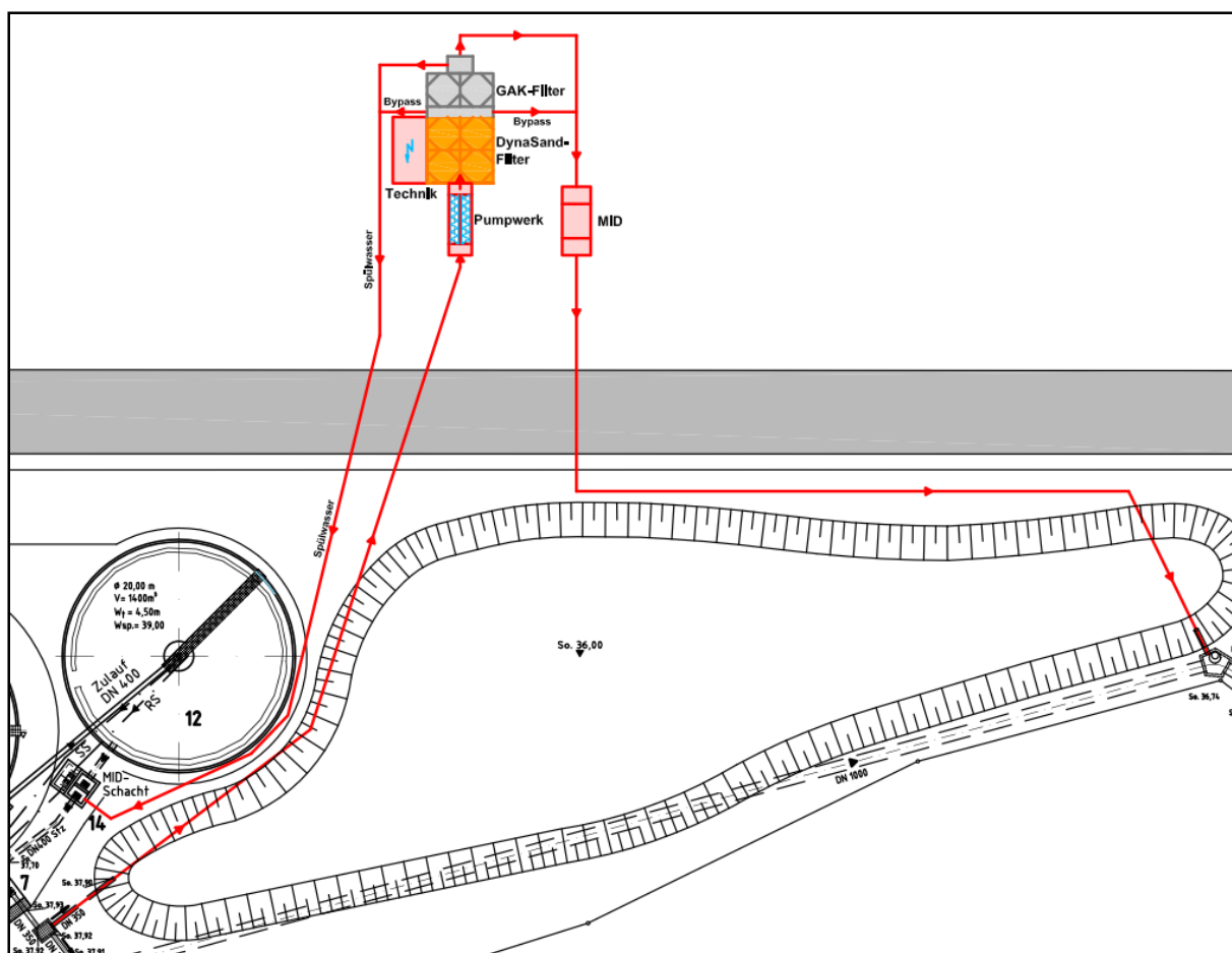
Abbildung 9.7: Mögliche Ausführungsform der Variante 2
