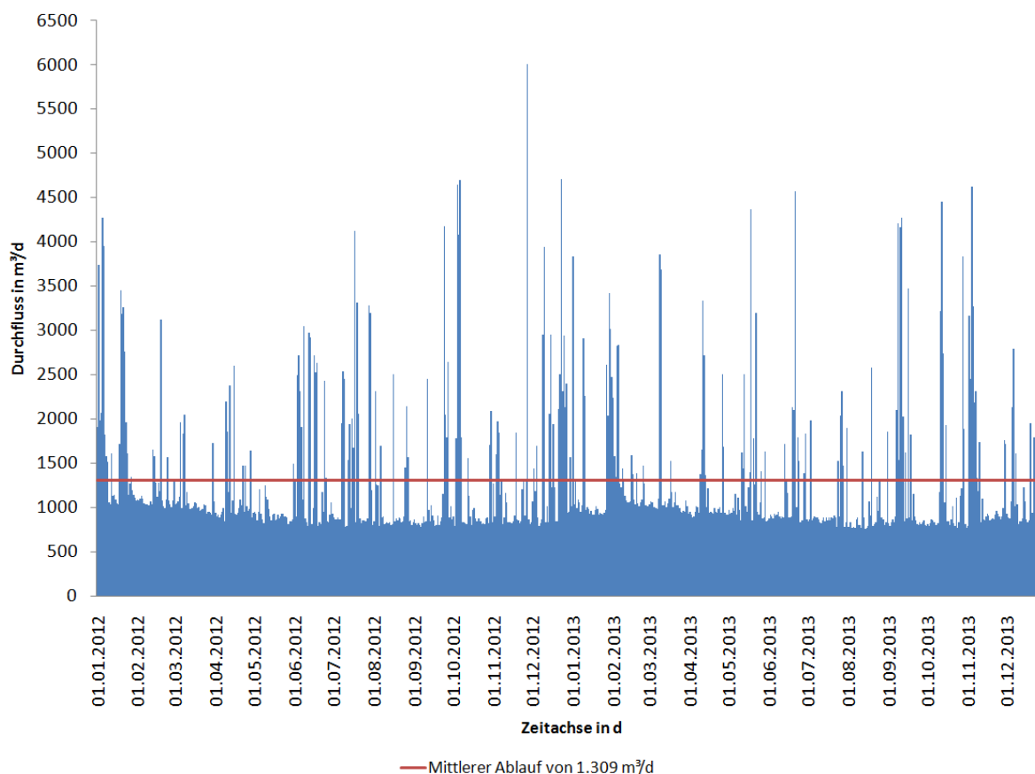
Abbildung 7.2: Ablaufmengen der Kläranlage Saerbeck im Zeitraum vom 01.01.2012 bis 31.12.2013
