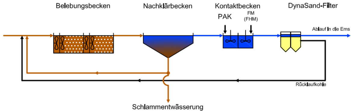
Abbildung 9.4: Fließschema der Variante 1.2
