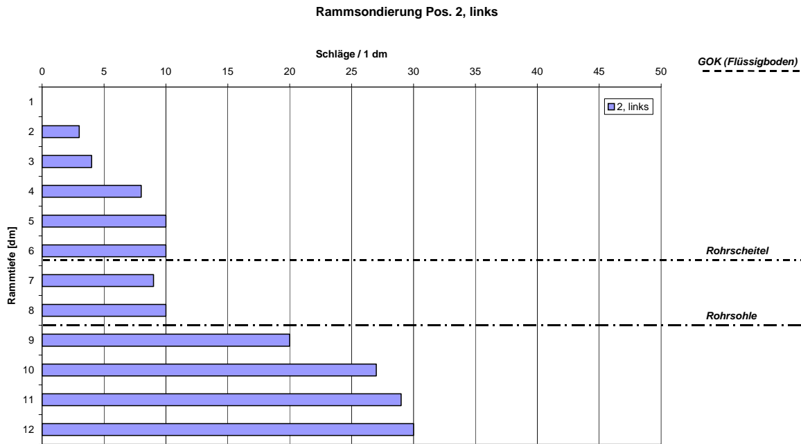
Bild 9: Versuch 2: Ergebnisse der Rammsondierung an Position 2, links
