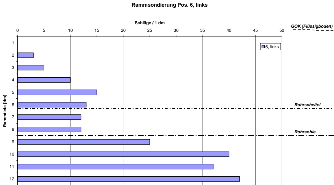
Bild 37: Versuch 4: Ergebnisse der Rammsondierung an Position 6, links
