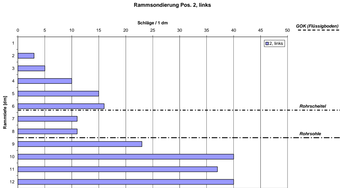
Bild 33: Versuch 4: Ergebnisse der Rammsondierung an Position 2, links
