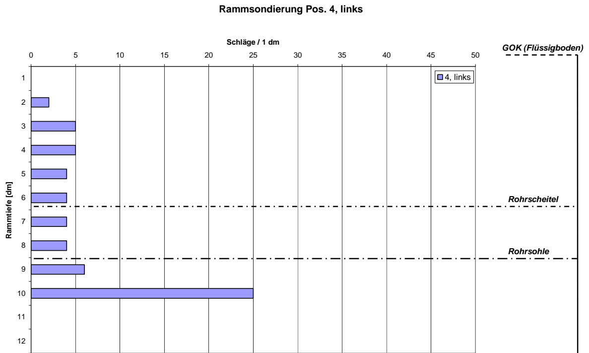
Bild 59: Versuch 7: Ergebnisse der Rammsondierung an Position 4, links
