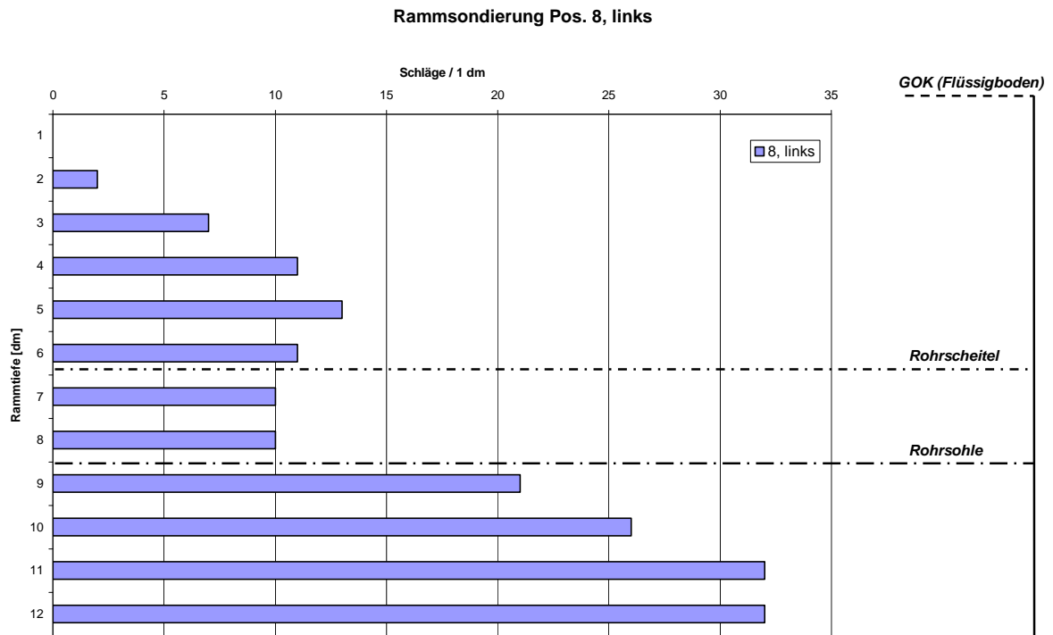
Bild 7: Versuch 1: Ergebnisse der Rammsondierung an Position 8, links
