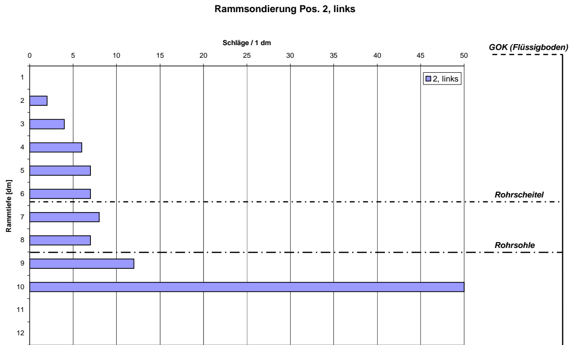
Bild 79: Versuch 9: Ergebnisse der Rammsondierung an Position 2, links
