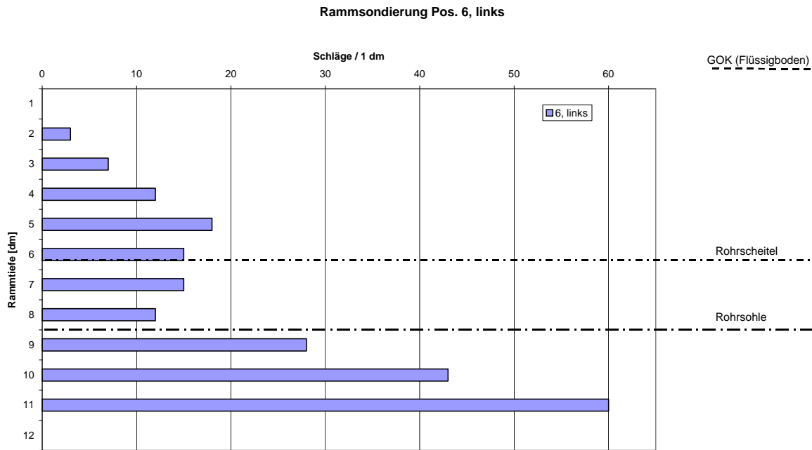
Bild 45: Versuch 5: Ergebnisse der Rammsondierung an Position 6, links
