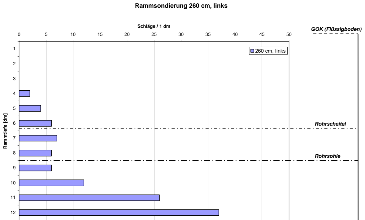
Bild 29: Versuch 3: Ergebnisse der Rammsondierung an Position 6, links
