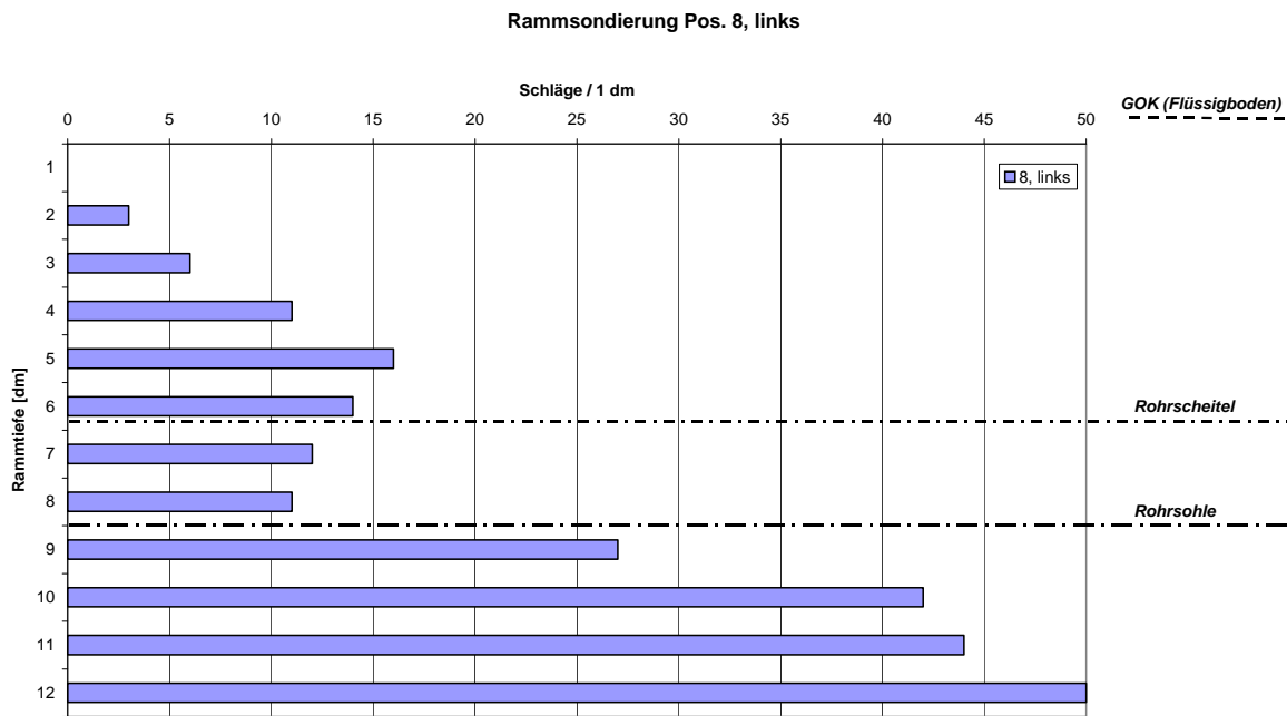
Bild 39: Versuch 4: Ergebnisse der Rammsondierung an Position 8, links
