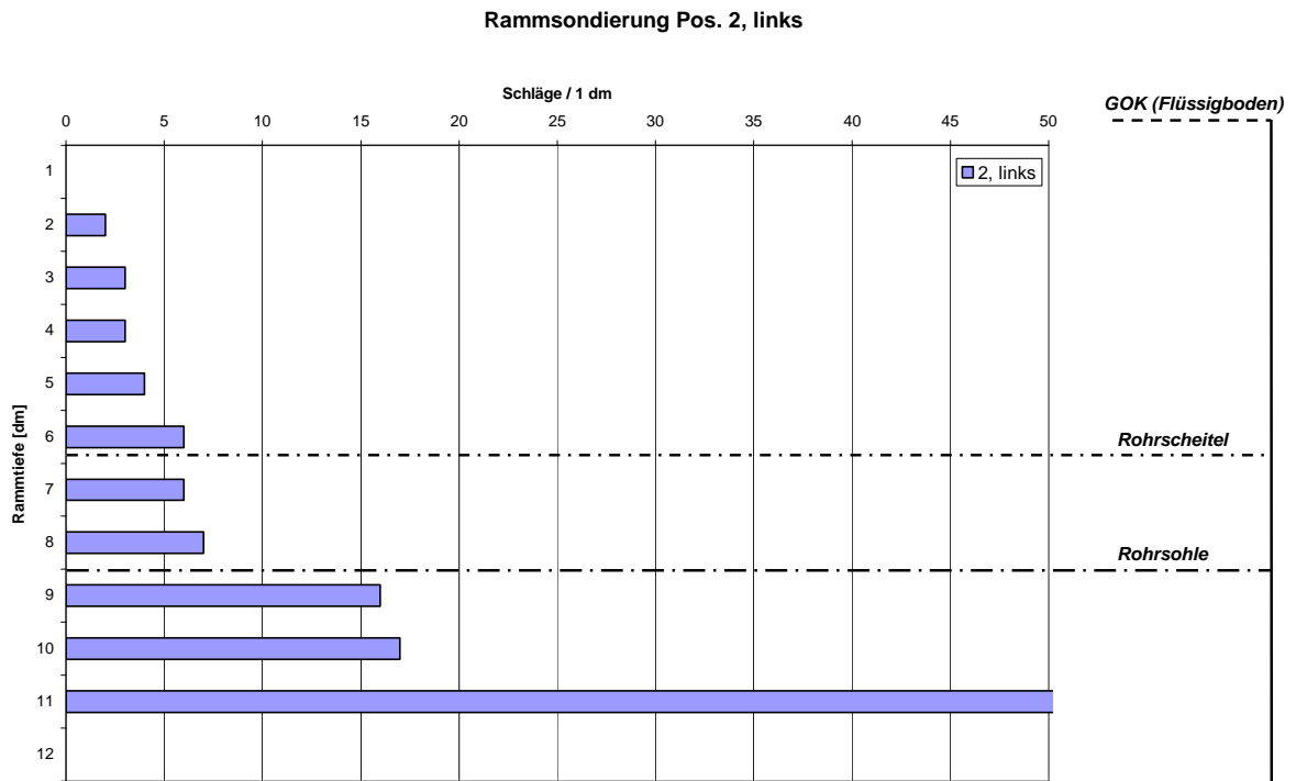
Bild 65: Ergebnisse der Rammsondierung für Versuch 8 an Position 2, links
