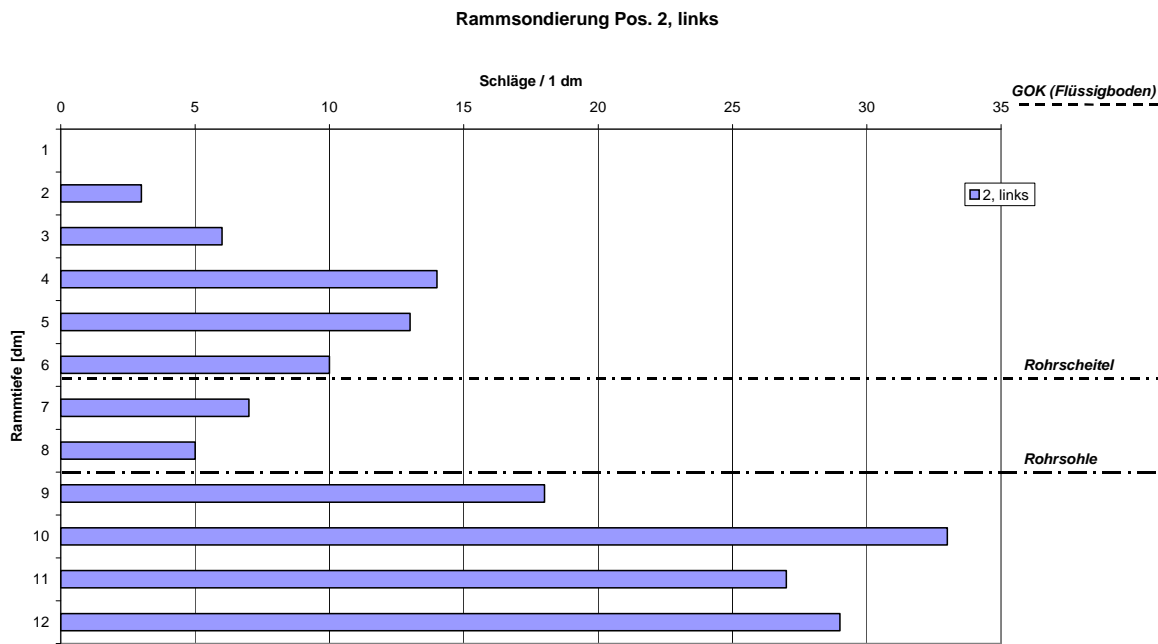
Bild 1: Versuch 1: Ergebnisse der Rammsondierung an Position 2, links
