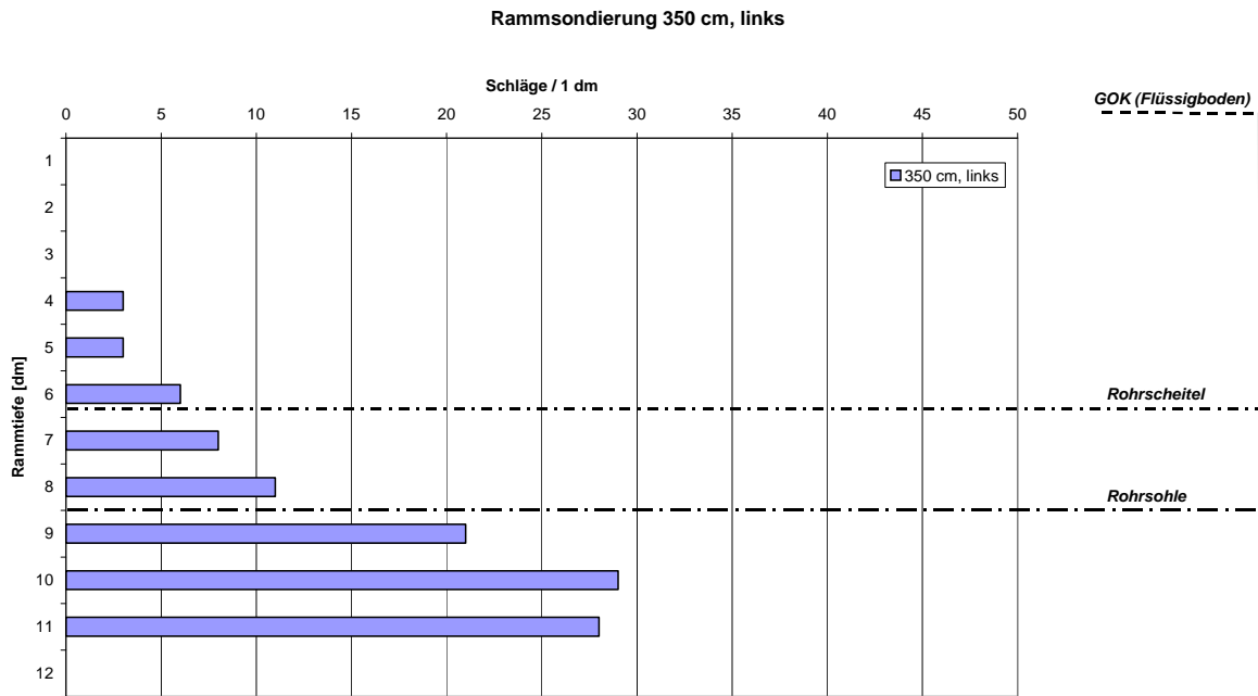
Bild 23: Versuch 3: Ergebnisse der Rammsondierung an Position 8, links, nur Innenverdichter
