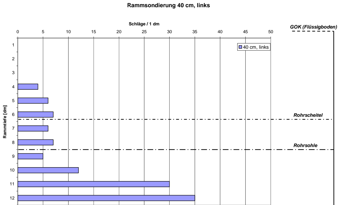
Bild 25: Versuch 3: Ergebnisse der Rammsondierung an Position 2, links
