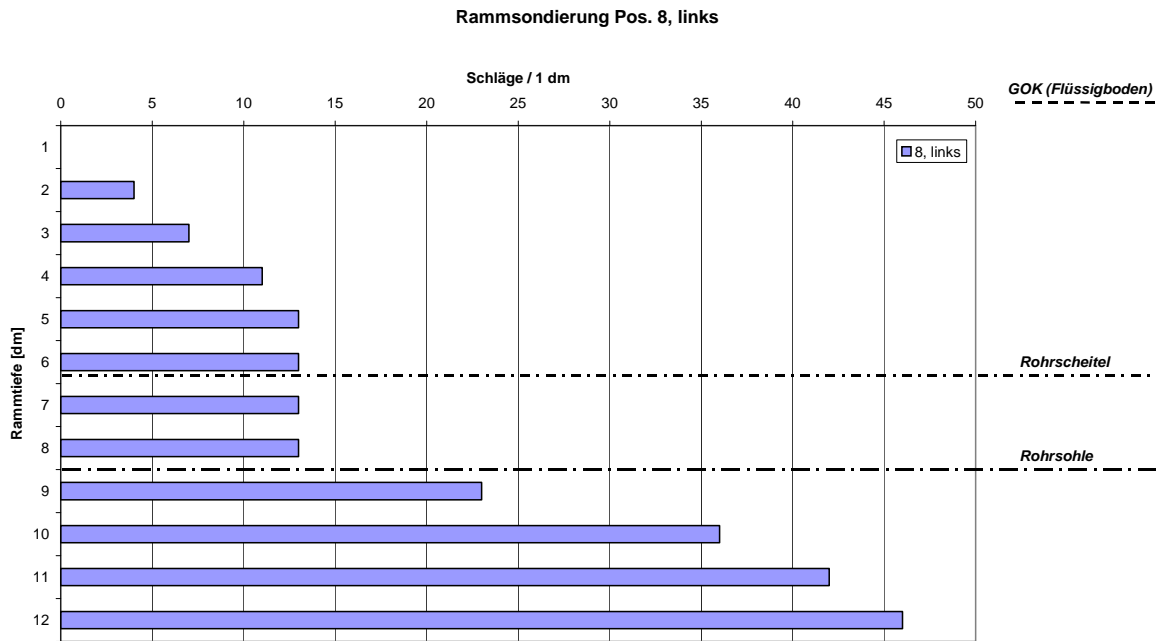
Bild 15: Versuch 2: Ergebnisse der Rammsondierung an Position 8, links
