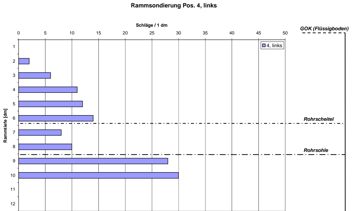
Bild 51: Versuch 6: Ergebnisse der Rammsondierung an Position 4, links
