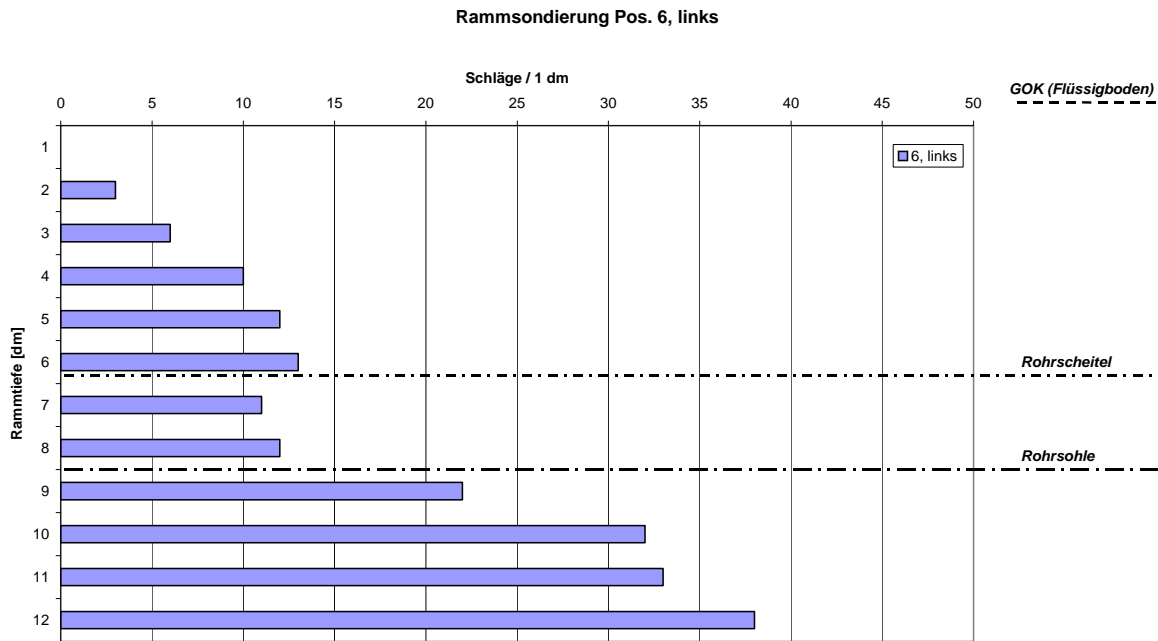
Bild 13: Versuch 2: Ergebnisse der Rammsondierung an Position 6, links
