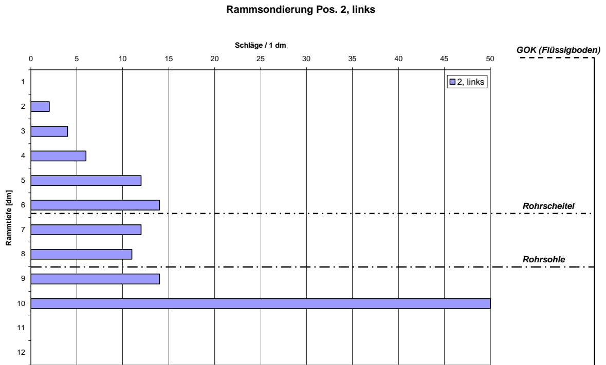
Bild 87: Versuch 10: Ergebnisse der Rammsondierung an Position 2, links
