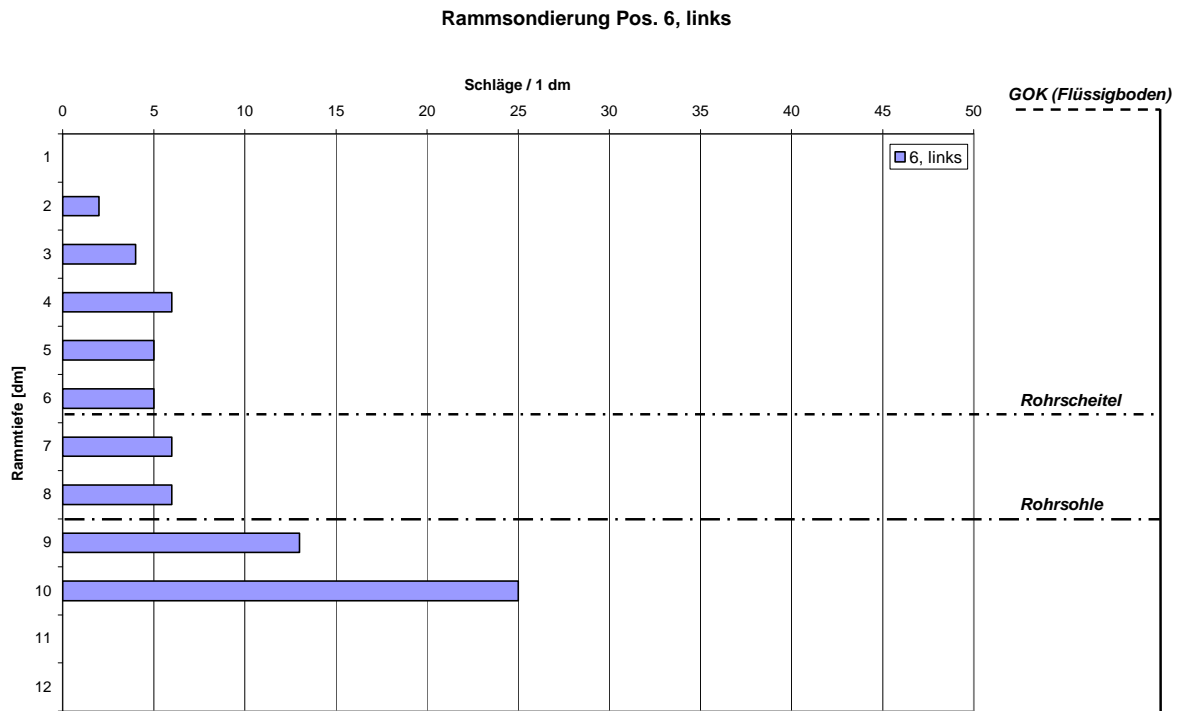
Bild 61: Versuch 7: Ergebnisse der Rammsondierung an Position 6, links
