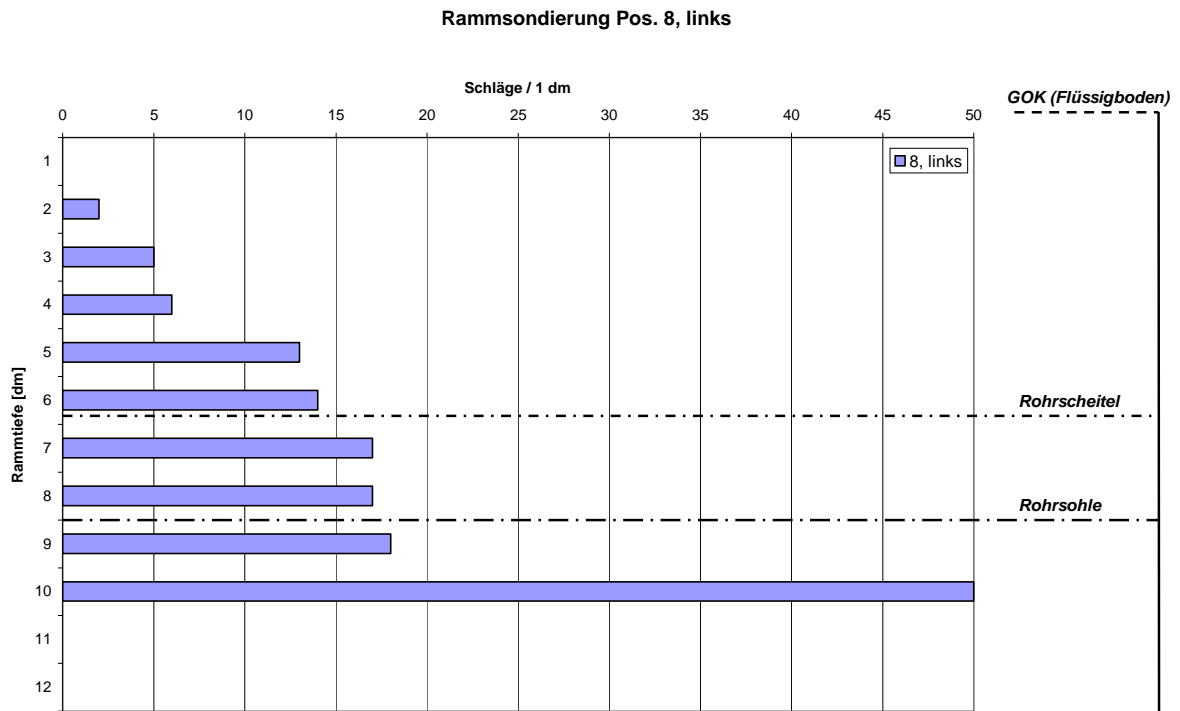
Bild 93: Versuch 10: Ergebnisse der Rammsondierung an Position 8, links
