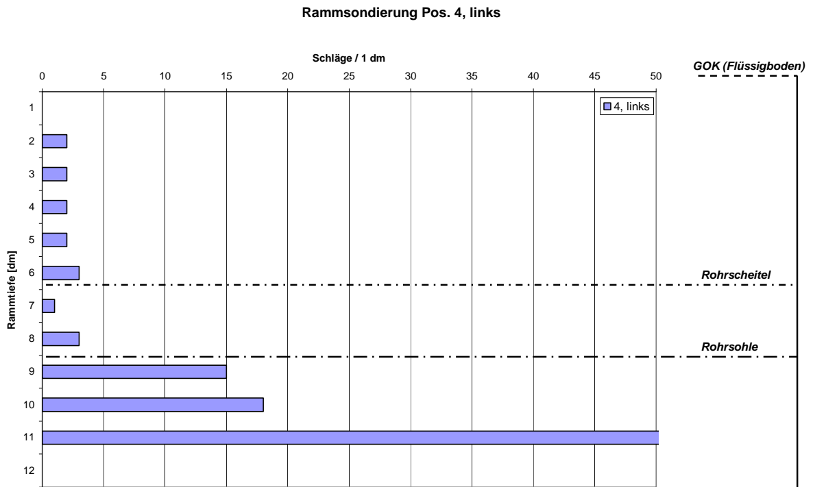
Bild 67: Versuch 8: Ergebnisse der Rammsondierung an Position 4, links
