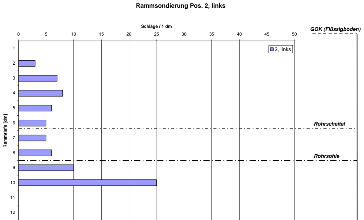
Bild 57: Versuch 7: Ergebnisse der Rammsondierung an Position 2, links
