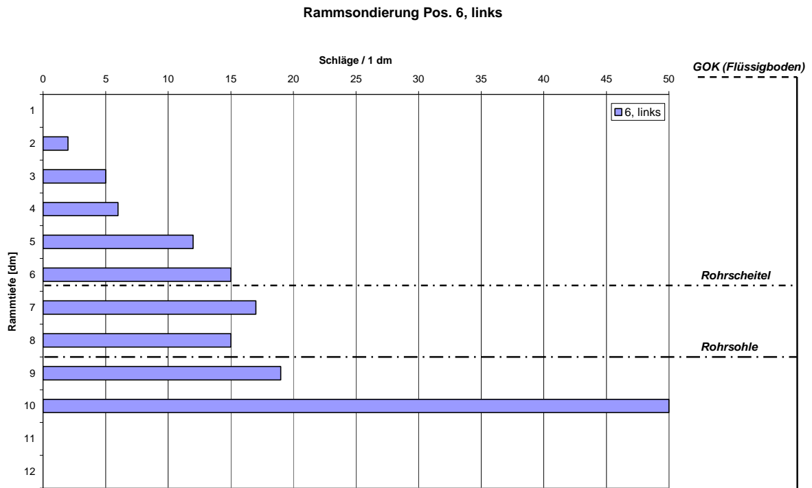
Bild 91: Versuch 10: Ergebnisse der Rammsondierung an Position 6, links
