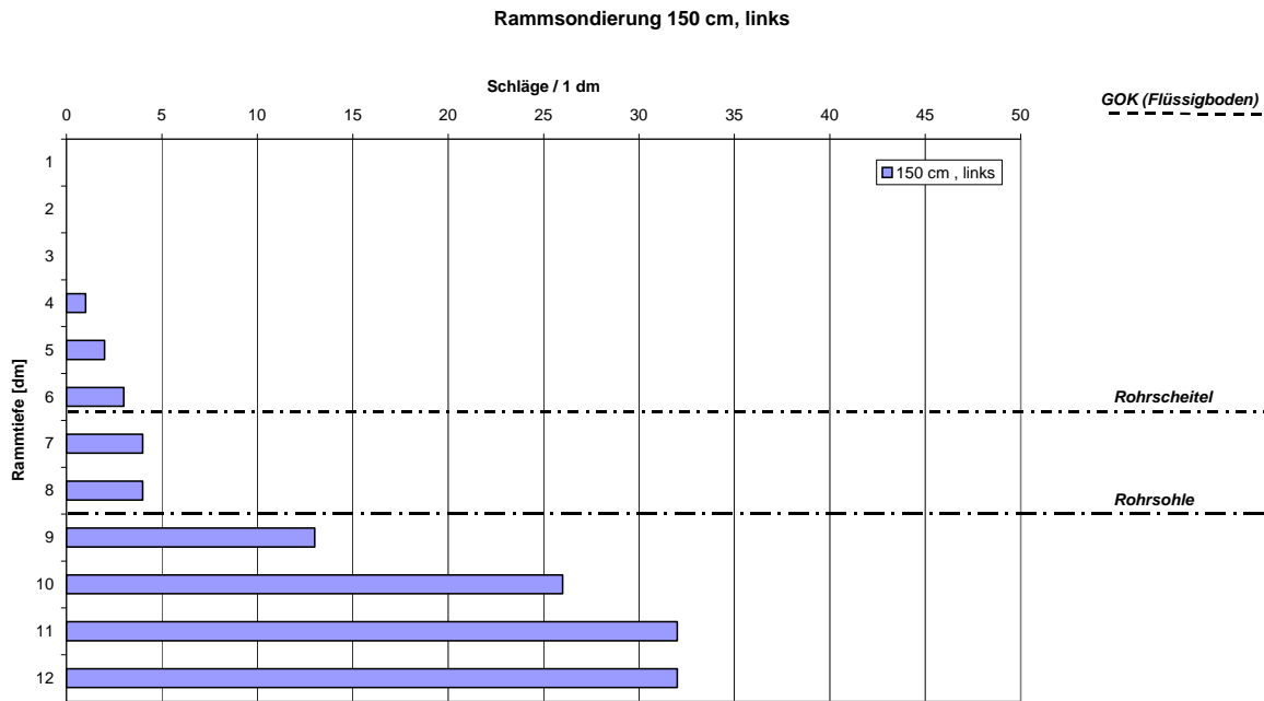
Bild 19: Versuch 3: Ergebnisse der Rammsondierung an Position 4, links, nur Innenverdichter
