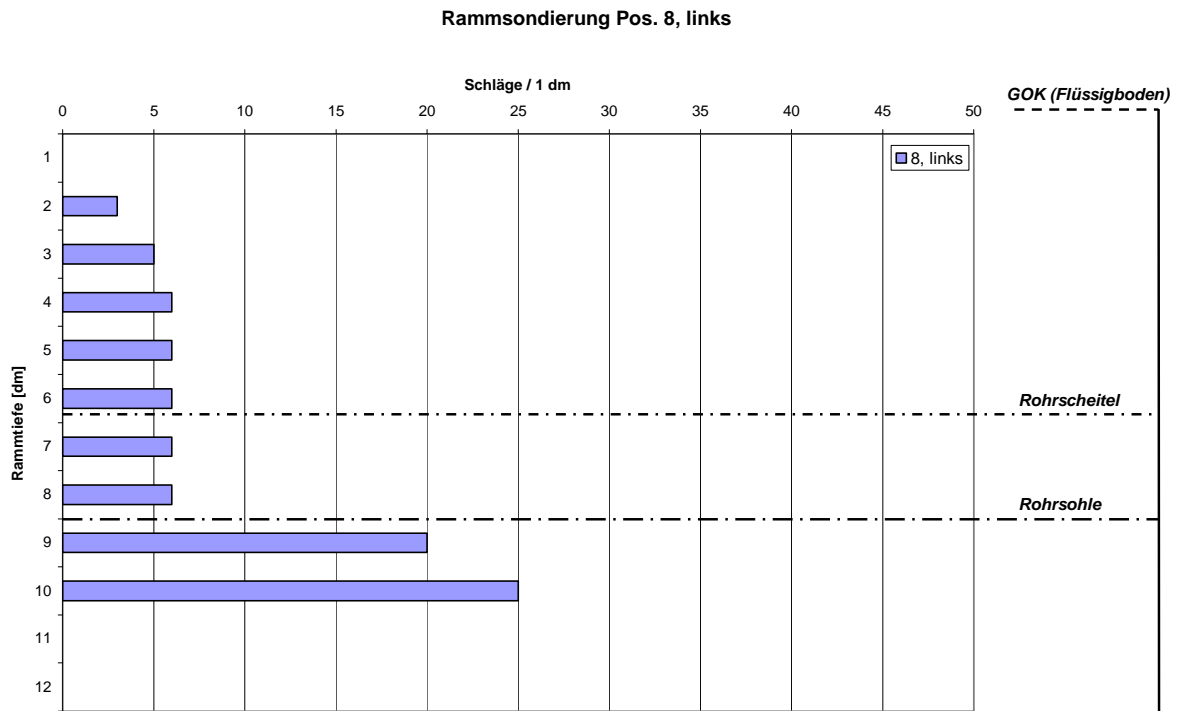
Bild 63: Versuch 7: Ergebnisse der Rammsondierung an Position 8, links
