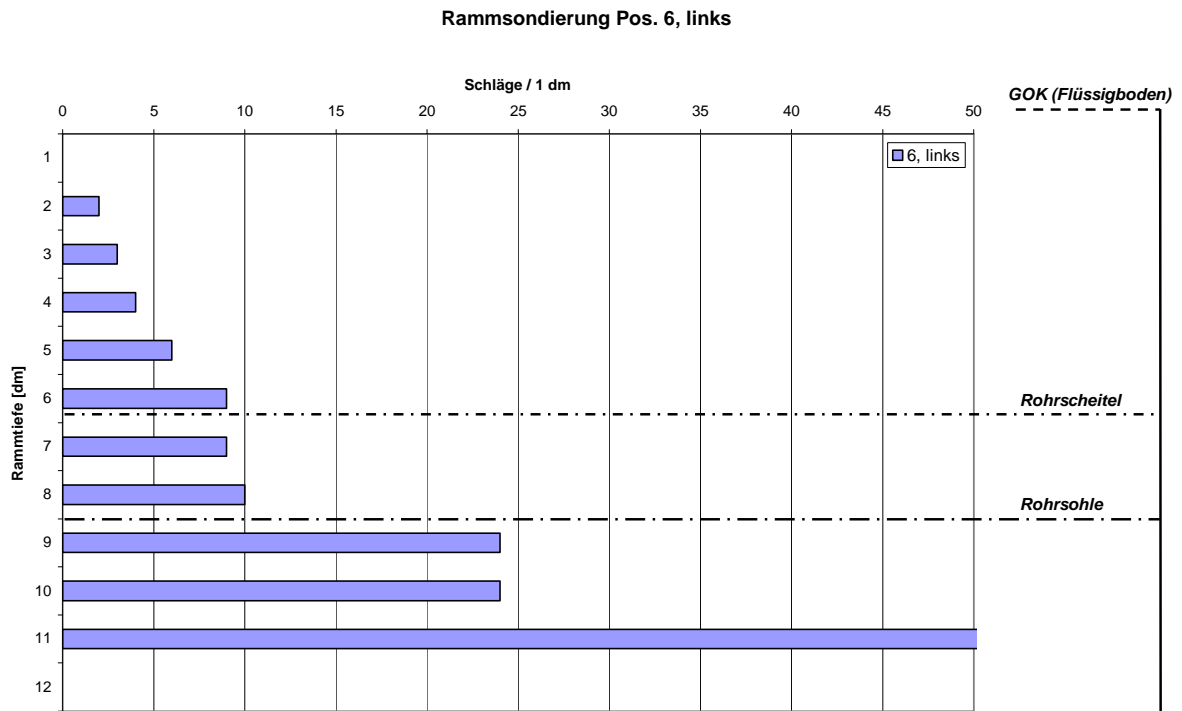
Bild 69: Versuch 8: Ergebnisse der Rammsondierung an Position 6, links
