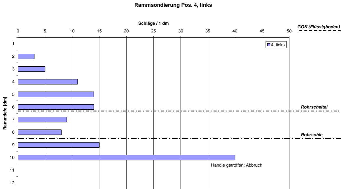
Bild 35: Versuch 4: Ergebnisse der Rammsondierung an Position 4, links
