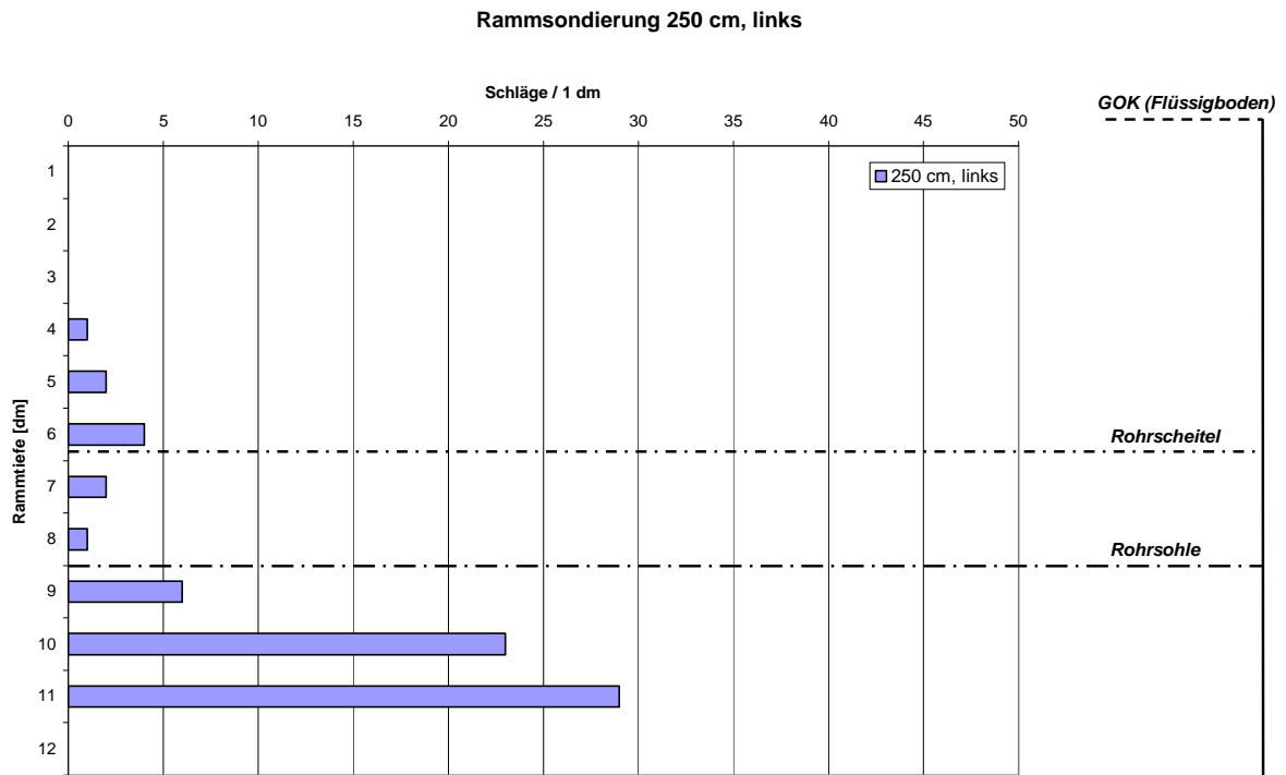
Bild 21: Versuch 3: Ergebnisse der Rammsondierung an Position 6, links, nur Innenverdichter
