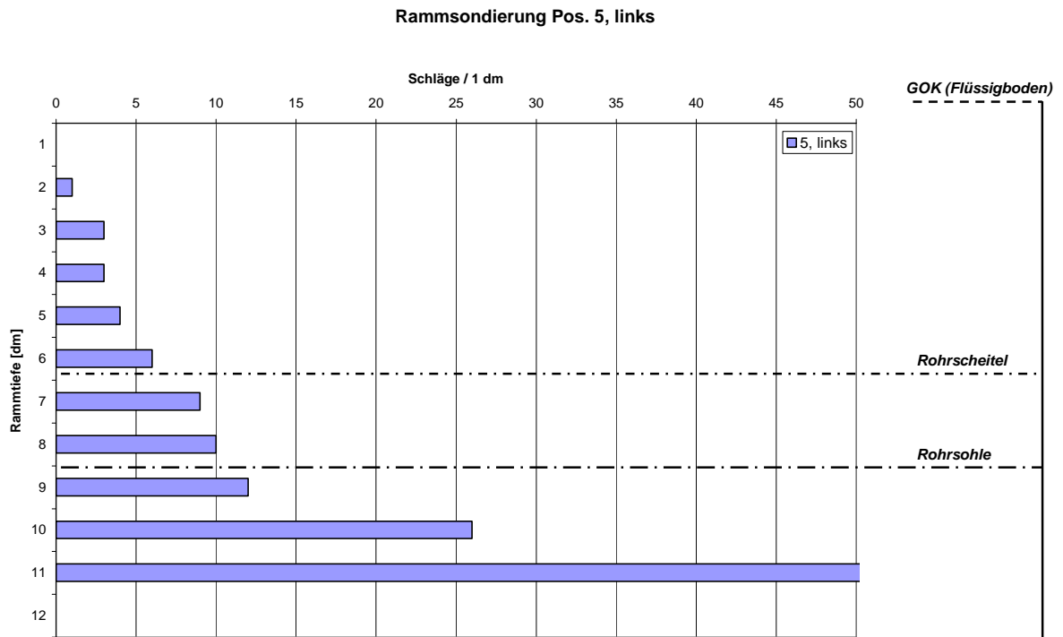
Bild 75: Versuch 8: Ergebnisse der Rammsondierung an Position 5, links
