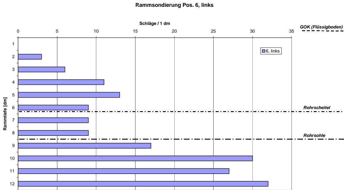
Bild 5: Versuch 1: Ergebnisse der Rammsondierung an Position 6, links
