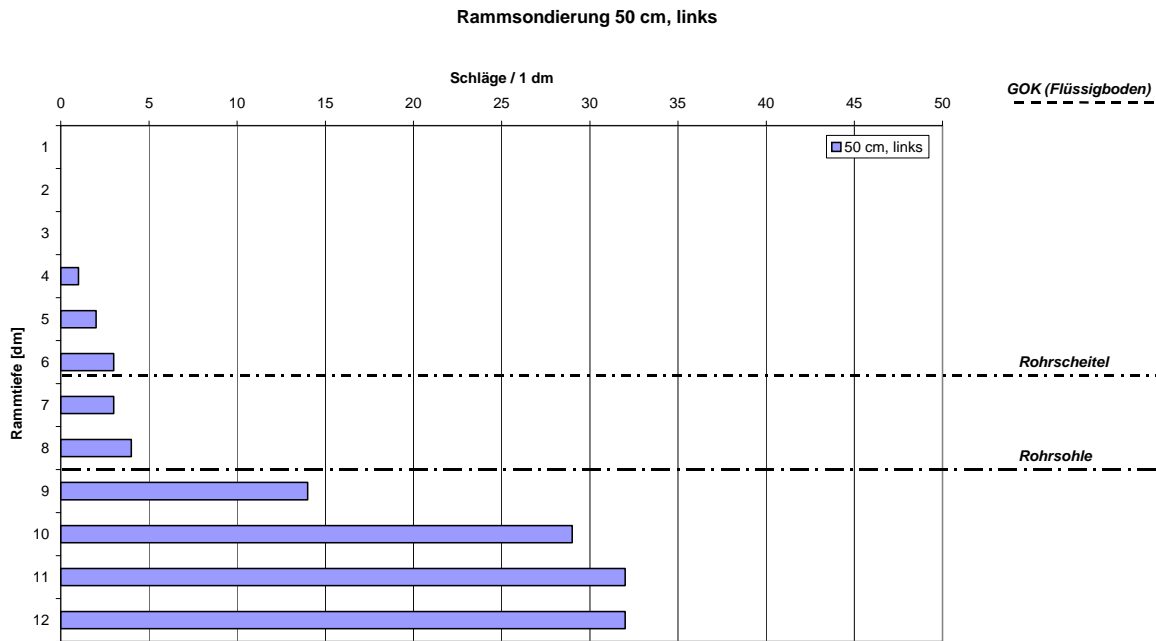
Bild 17: Versuch 3: Ergebnisse der Rammsondierung an Position 2, links, nur Innenverdichter
