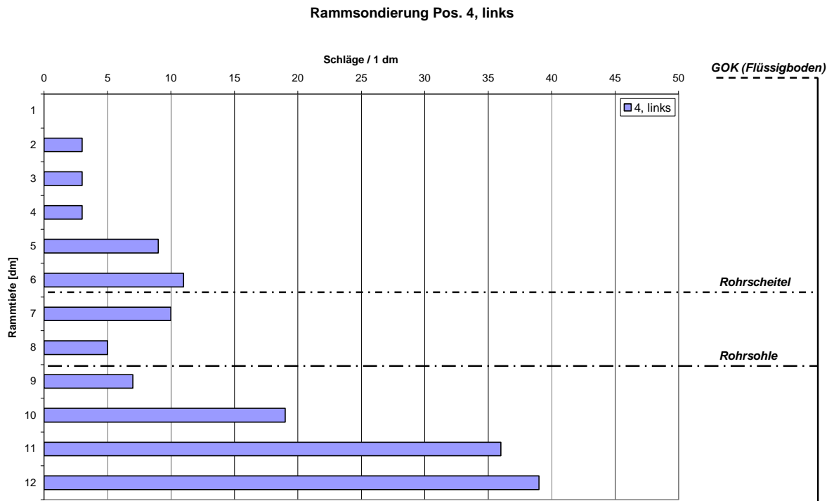
Bild 11: Versuch 2: Ergebnisse der Rammsondierung an Position 4, links
