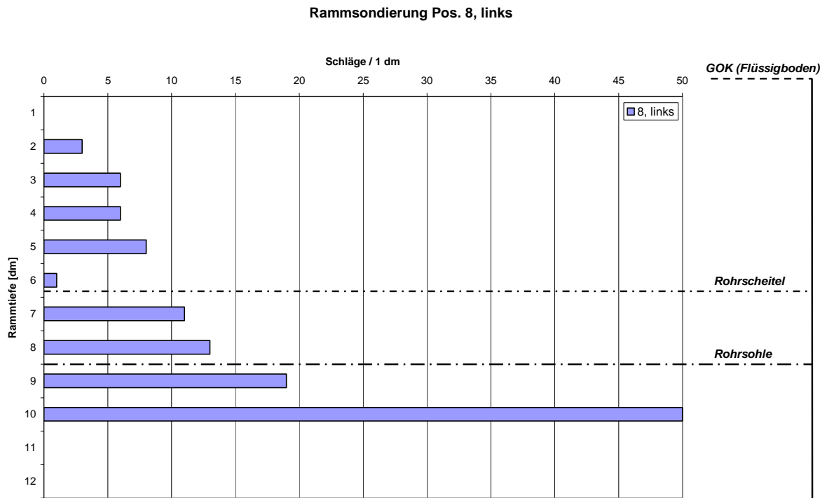
Bild 85: Versuch 9: Ergebnisse der Rammsondierung an Position 8, links
