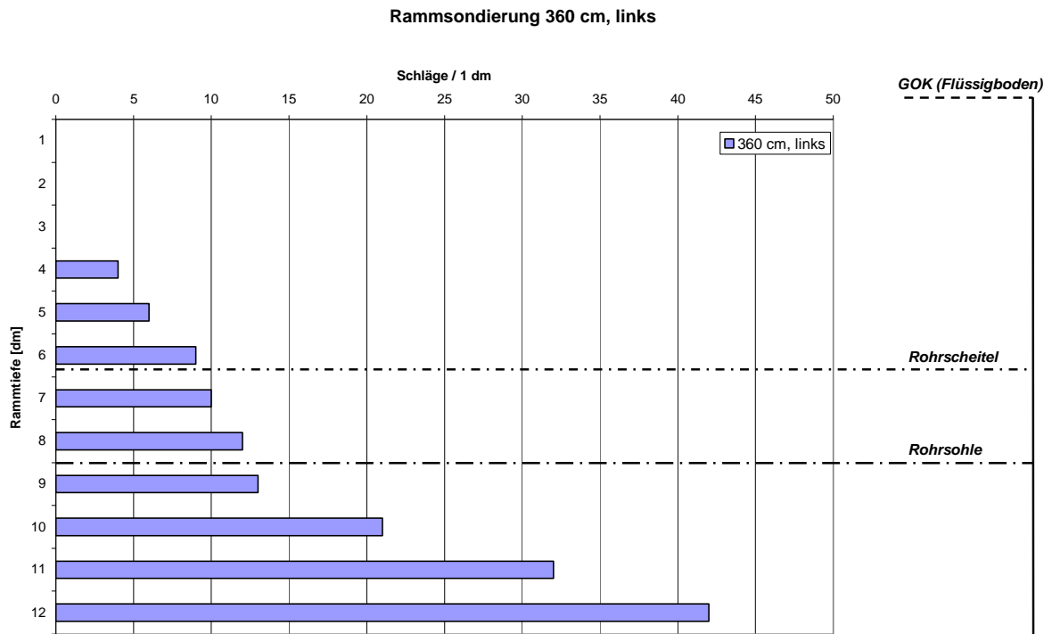
Bild 31: Versuch 3: Ergebnisse der Rammsondierung an Position 8, links
