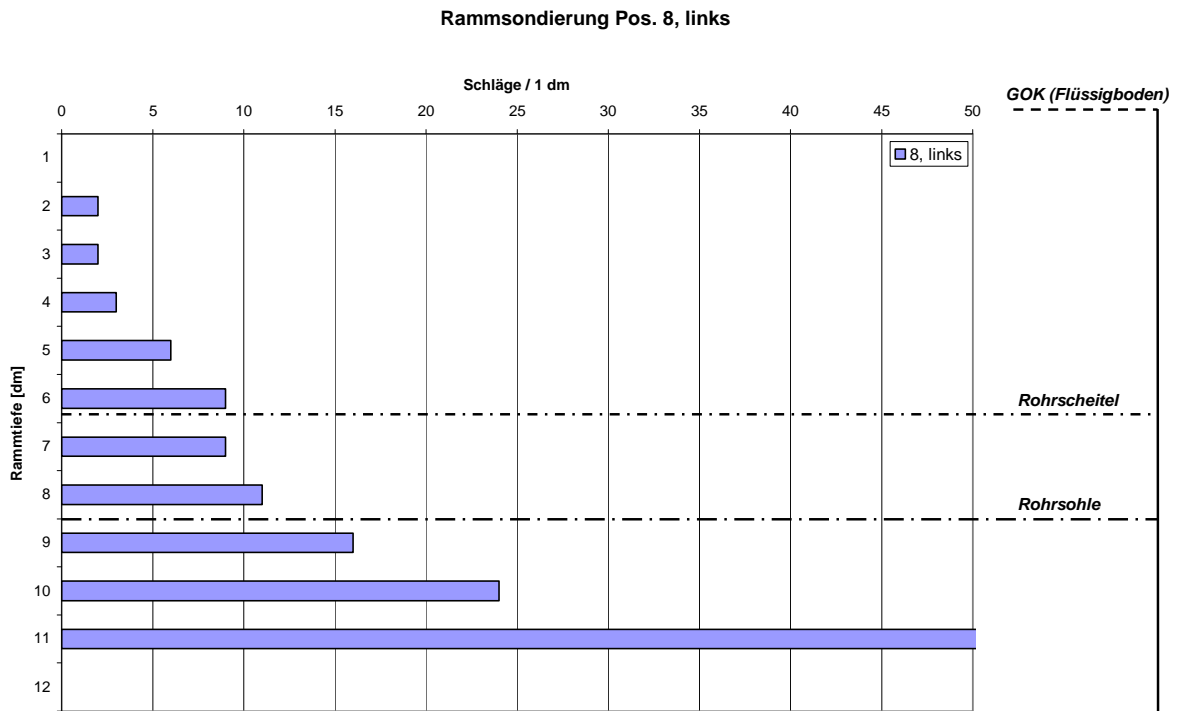
Bild 71: Versuch 8: Ergebnisse der Rammsondierung an Position 8, links
