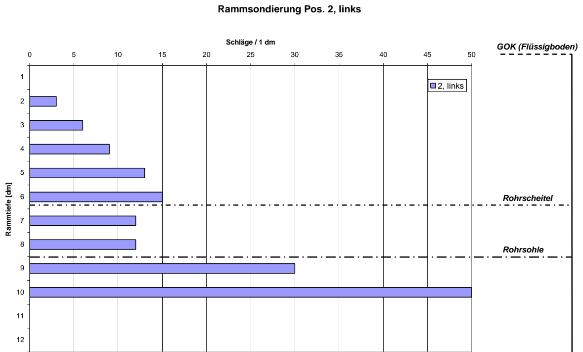
Bild 49: Versuch 6: Ergebnisse der Rammsondierung an Position 2, links
