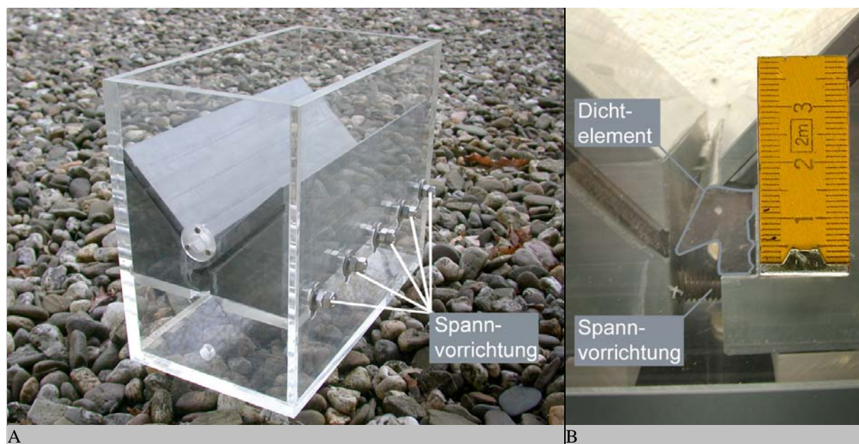
Abb. 98: Untersuchung des Wurzelwachstums an elastomeren Dichtelementen. A Seitenansicht der Vorrichtung. B Detail eines eingebauten Dichtungselementes. Der Querschnitt des Dichtelementes wurde für die Abbildung hervorgehoben.
