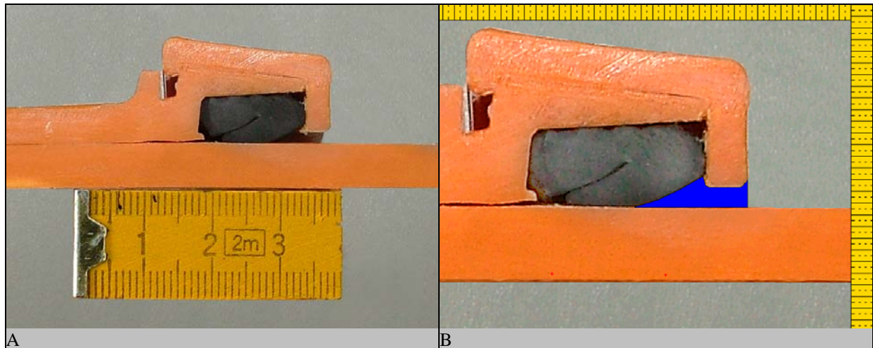
Abb. 111: Untersuchung der Verbindungsgeometrie. Rohrverbindung Rausisto SN 10 PP, DN/OD 160. A Längsschnitt durch die Rohrverbindung. B Detail Dichtelement. Ringspalt = 0,3 mm. Der blau gekennzeichnete Raum vor dem Dichtelement hat eine Fläche von 14 mm 2 .
