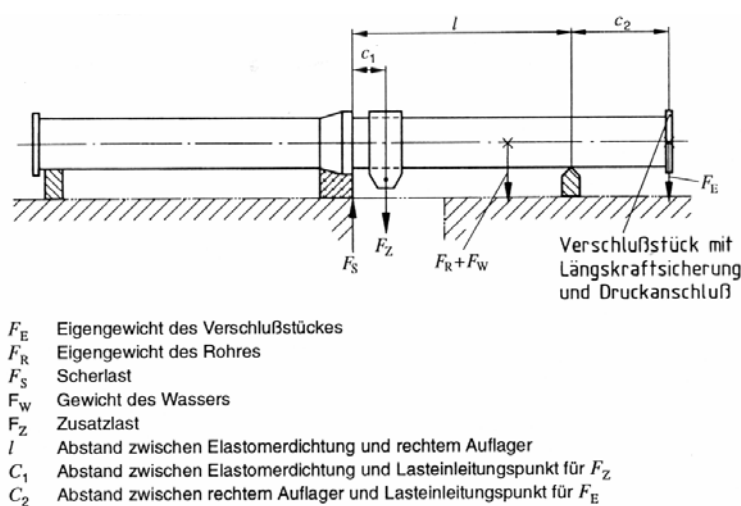
Abb. 6: Scherlastprüfung nach DIN 4060 [4].
