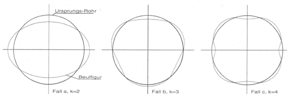
Abb. 39 Darstellung von zwei- drei- sowie vierwelligen Beulfiguren [65]
