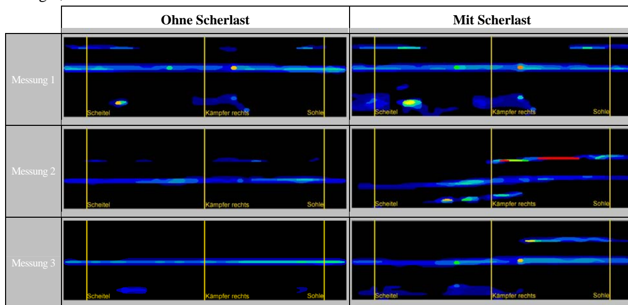
Abb. 29: Messung des Anpressdruckes mittels einer Druckfolie. Rohrverbindung Rehau Awadukt SN4 PVC DN/OD 160 ohne Scherlast und mit Scherlast nach DIN [4]. Maßgeblicher Anpressdruck im Bereich der Rohrsohle: Messung 1) ohne Scherlast-Wirkung 10,7 bar, mit Scherlast-Wirkung 9,0 bar Messung 2) ohne Scherlast-Wirkung 4,5 bar, mit Scherlast-Wirkung 2,4 bar, Messung 3) ohne Scherlast-Wirkung 8,1 bar, mit Scherlast-Wirkung 7,5 bar. Mittelwerte des Anpressdruckes ohne Scherlast 7,7 bar , mit Scherlast 6,3 bar .
