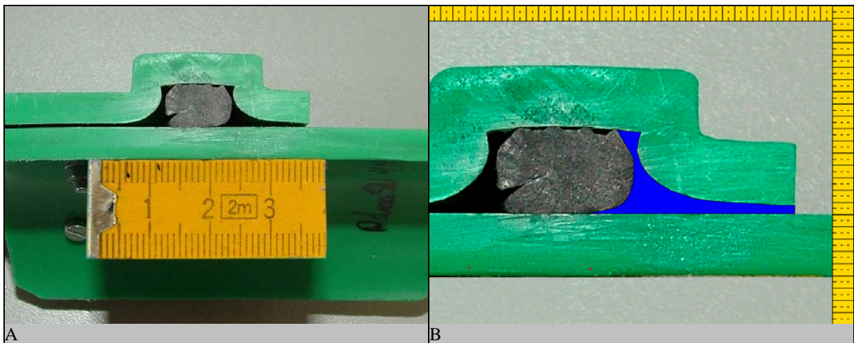
Abb. 110: Untersuchung der Verbindungsgeometrie. Rohrverbindung Rehau Awadukt SN4 PP. A Längsschnitt durch die Rohrverbindung. B . Detail Dichtelement. Ringspalt = 0,6 mm. Der blau gekennzeichnete Raum vor dem Dichtelement hat eine Fläche von 28 mm 2 .
