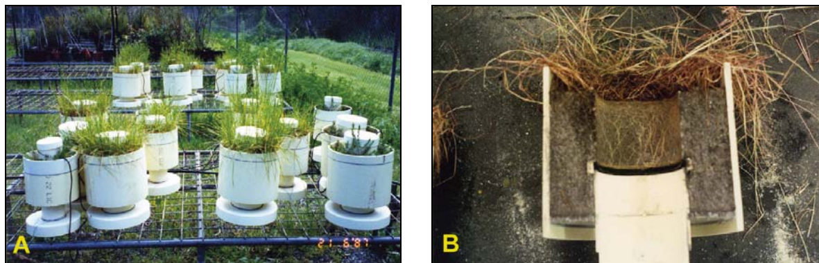
Abb. 16: Vertikale Versuche des CSIRO, Australien: A Rohrverbindungen im bepflanzten Zustand. B Rohrverbindung nach dem Ausbau, längs aufgeschnitten [54].
