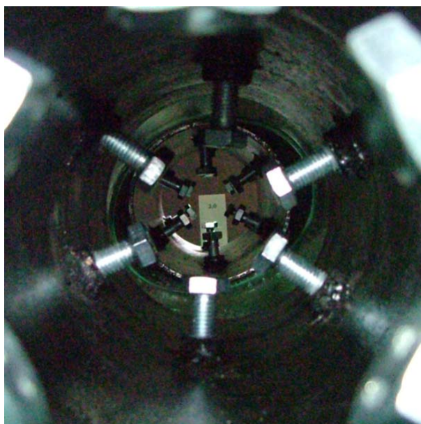
Abb.78: Rohrverbindung Rehau Awadukt PP SN 4 bei einem Außenüberdruck von 3,0 bar. Kein Wassereintritt.
