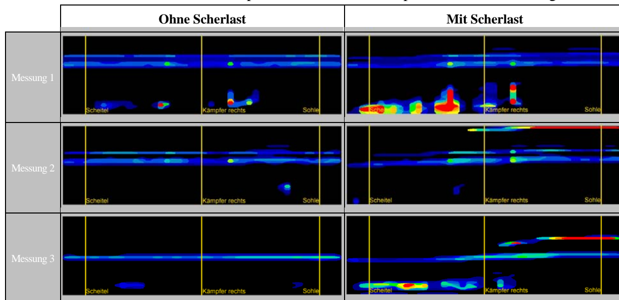
Abb. 28: Messung des Anpressdruckes mittels einer Druckfolie. Rohrverbindung Ostendorf KG PVC DN 160 ohne Scherlast und mit Scherlast nach DIN [4]. Maßgeblicher Anpressdruck im Bereich der Rohrsohle: Messung 1) ohne Scherlast-Wirkung 4,4 bar, mit Scherlast-Wirkung 3,1 bar Messung 2) ohne Scherlast-Wirkung 4,4 bar, mit Scherlast-Wirkung 2,9 bar, Messung 3) ohne Scherlast-Wirkung 4,8 bar, mit Scherlast-Wirkung 3,3 bar. Mittelwerte des Anpressdruckes ohne Scherlast 4,5 bar , mit Scherlast 3,1 bar .
