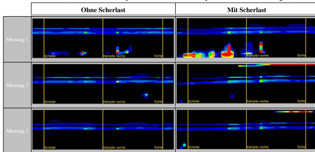
Abb. 32: Messung des Anpressdruckes mittels einer Druckfolie. Rohrverbindung Ostendorf KG-2000, DN 150 ohne Scherlast und mit Scherlast nach DIN [4]. Maßgeblicher Anpressdruck im Bereich der Rohrsohle: Messung 1) ohne Scherlast-Wirkung 4,7 bar, mit Scherlast-Wirkung 1,2 bar Messung 2) ohne Scherlast-Wirkung 3,5 bar, mit Scherlast-Wirkung 2,5 bar, Messung 3) ohne Scherlast-Wirkung 4,3 bar, mit Scherlast-Wirkung 4,5 bar. Mittelwerte des Anpressdruckes ohne Scherlast 4,1 bar , mit Scherlast 2,7 bar .
