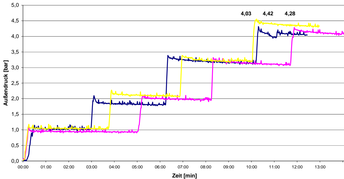
Abb. 70: Ergebnisse der Außenüberdruckuntersuchungen an Rohrverbindungen vom Typ Awadukt PVC SN8. Im Diagramm sind die Messwerte dreier Messungen aufgetragen. Die Höchstwerte geben den Höchstdruck des Wasserversorgungsnetzes wieder.
