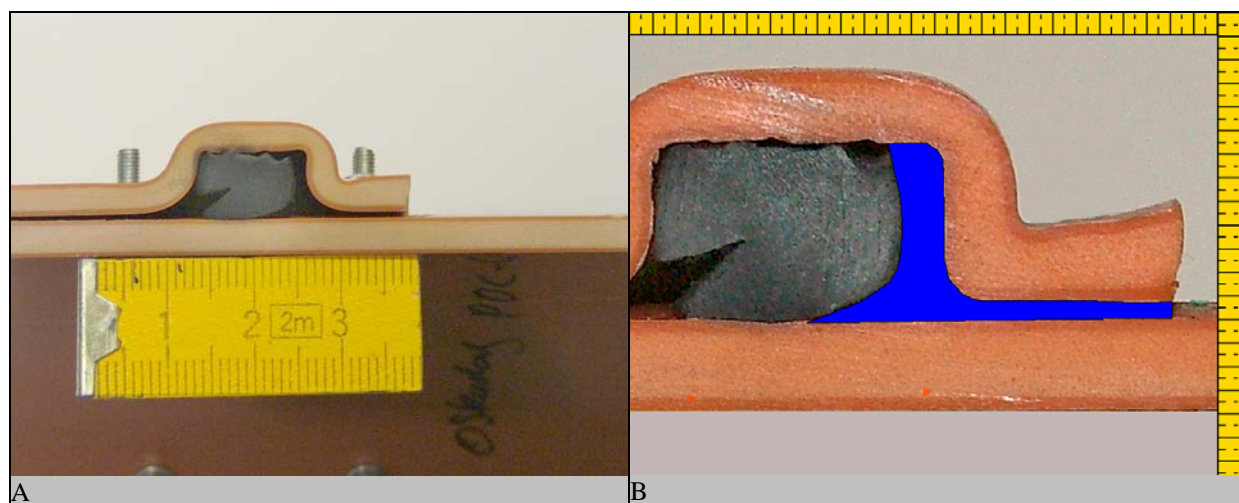
Abb. 105: Untersuchung der Verbindungsgeometrie. Rohrverbindung Ostendorf KG-PVC DN 160. A Längsschnitt durch die Rohrverbindung. B Detail des Dichtelementes. Ringspalt = 0,7 mm. Der blau gekennzeichnete Raum vor dem Dichtelement hat im Längsschnitt eine Fläche von 38 mm 2 .
