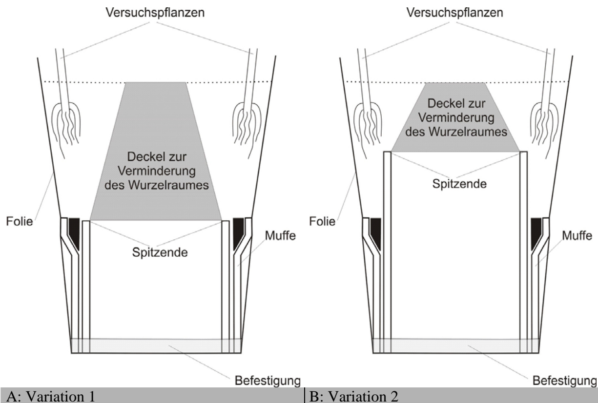
Abb. 91: Längsschnitt der Kulturgefäße für die Outside-In-Versuche. Zur Verminderung des Wurzelraumes und der Versuchsdauer wurde eine Abdeckung oberhalb des Spitzendes angebracht. A Beispiel eines Kulturgefäßes, bei dem Spitzende und Muffe bündig abschließen, im weiteren auch als „Variation 1“ bezeichnet. B Beispiel eines Kulturgefäßes, bei dem ein Trichtereffekt eintritt, durch den die Wurzeln in Richtung des Dichtelements geleitet werden können, im weiteren auch als „Variation 2“ bezeichnet.
