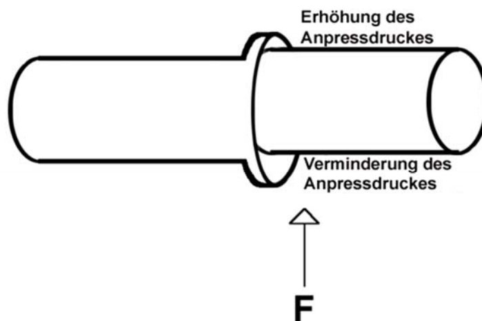
Abb. 20: Wirkung der Scherlast auf den Anpressdruck des Dichtelementes einer Rohrverbindung. Verminderung des Anpressdruckes im Bereich der Sohle, Erhöhung des Anpressdruckes im Bereich des Scheitels.
