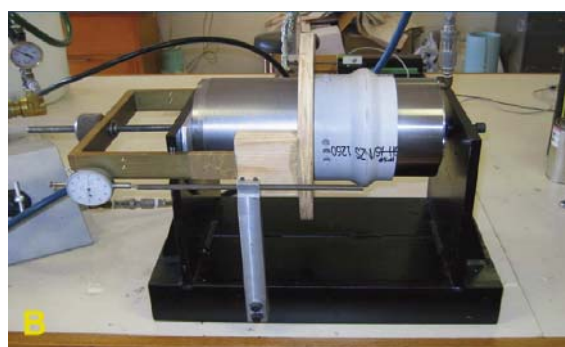
Abb. 15: Bestimmung des Anpressdrucks in der Rohrverbindung nach AS 1462 Part 13: A Schematische Darstellung des Versuchsaufbaus (vgl. [54]). B Versuchsstand mit Weg- und Druckmессeinrichtung (vgl. [54]).
