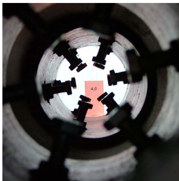
Abb.69: Rohrverbindung Awadukt PVC SN8, bei einem Außenüberdruck von 4,0 bar. Kein Wassereintritt.
