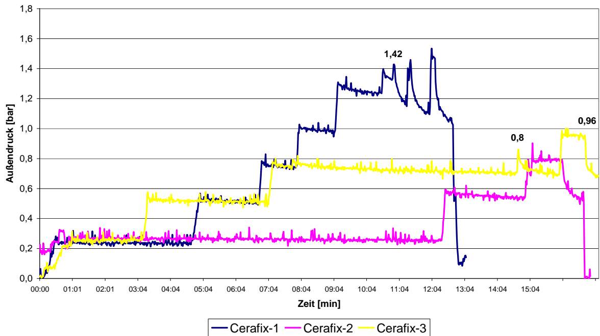
Abb. 43: Ergebnisse der Außendruckuntersuchungen an Rohrverbindungen vom Typ Steinzeug Cerafix DN150. Im Diagramm sind die Messwerte dreier Messungen aufgetragen. Die eingetragenen Werte geben den jeweiligen Versagensdruck für die entsprechenden Rohrverbindungen wieder.
