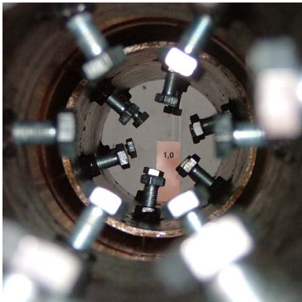
Abb.61: Rohrverbindung Wavin KG PVC bei einem Außenüberdruck von 1,0 bar. Kein Wassereintritt.
