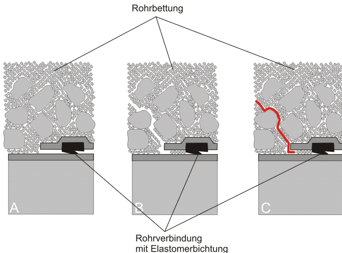
Abb. 3: Schematische Darstellung einer eingebauten Rohrverbindung (Steckverbindung) mit Elastomerichtung in ihrem Bettungsmaterial. A Zustand direkt nach dem Einbau. B mögliche Beeinträchtigung der Bodenstruktur durch Eindringen von Bodenpartikeln in den Ringspalt der Rohrverbindung zwischen Muffe und Spitze oder Setzungen durch nachträgliche Verdichtungen im Zwickelbereich der Leitung. Entstehung eines Dichtegradienten. C Möglicher Weg für einen Wurzeinwuchs durch die beeinträchtigte Bodenstruktur (rot).
