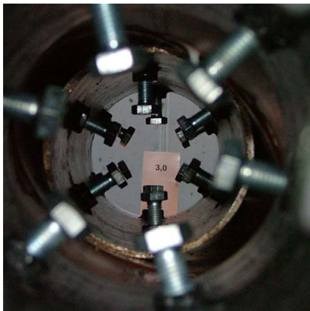
Abb.63: Rohrverbindung Wavin KG PVC bei einem Außenüberdruck von 3,0 bar. Kein Wassereintritt.
