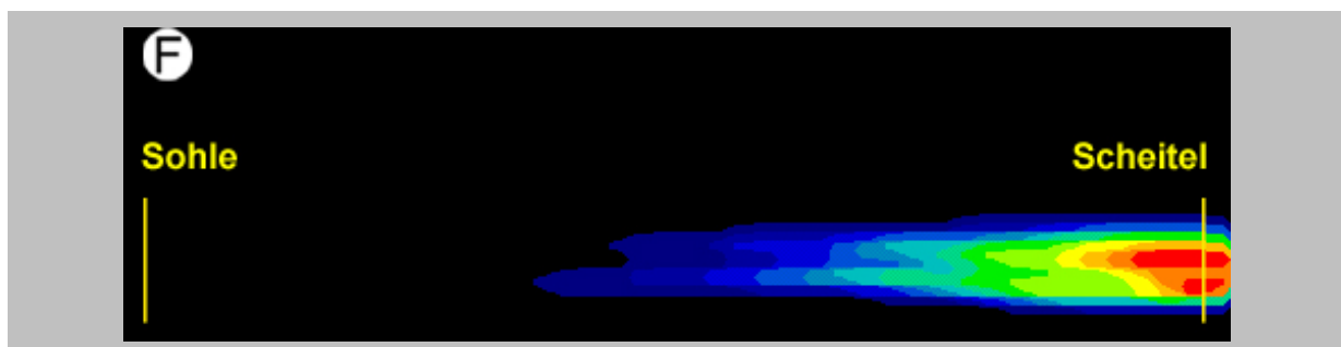
Abb. 23: Anpressdruckbild einer Rohrverbindung von der Rohrsohle bis zum Rohrscheitel unter Scherlast.
