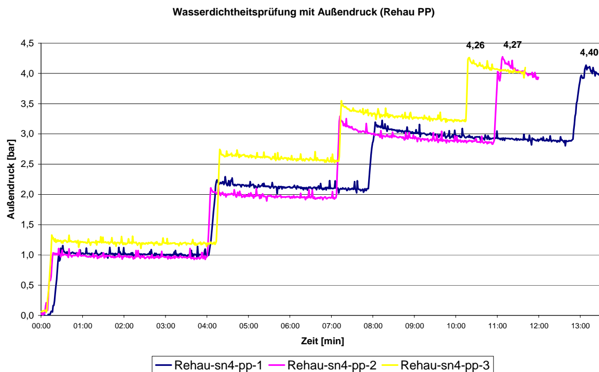
Abb. 80: Ergebnisse der Außendruckuntersuchungen an Rohrverbindungen vom Typ Rehau Awadukt SN 4 PP. Im Diagramm sind die Messwerte dreier Messungen aufgetragen. Die Höchstwerte geben den Höchstdruck des Wasserversorgungsnetzes wieder.
