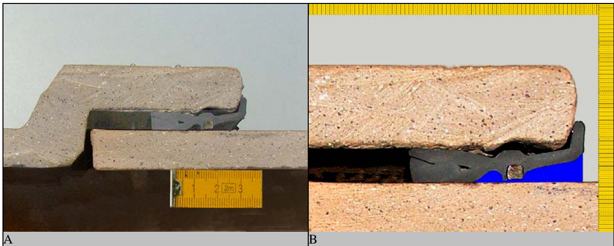
Abb. 103: Untersuchung der Verbindungsgeometrie. Rohrverbindung Euroceramic Eurotrade DN 150. A Längsschnitt durch die Rohrverbindung. B Detail des Dichtelementes. Ringspalt = 4,0 mm. Der blau gekennzeichnete Raum vor dem Dichtelement hat im Längsschnitt eine Fläche von 83 mm 2 .
