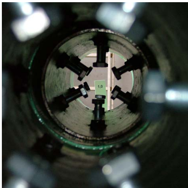
Abb.71: Rohrverbindung Ostendorf KG-2000 PP, bei einem Außenüberdruck von 1,0 bar. Kein Wassereintritt.
