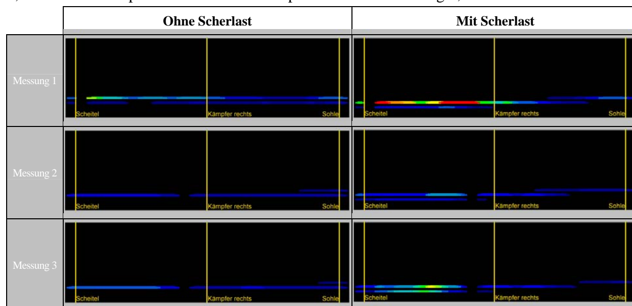
Abb. 27: Messung des Anpressdruckes mittels einer Druckfolie. Rohrverbindung Euroceramic/Hepworth Eurotop DN 150 ohne Scherlast und mit Scherlast nach DIN [4]. Maßgeblicher Anpressdruck im Bereich der Rohrsohle: Messung 1) ohne Scherlast-Wirkung 3,7 bar, mit Scherlast-Wirkung 4,3 bar Messung 2) ohne Scherlast-Wirkung 1,7 bar, mit Scherlast-Wirkung 1,5 bar, Messung 3) ohne Scherlast-Wirkung 2,0 bar, mit Scherlast-Wirkung 0,1 bar. Mittelwerte des Anpressdruckes ohne Scherlast 2,5 bar , mit Scherlast 2,0 bar .
