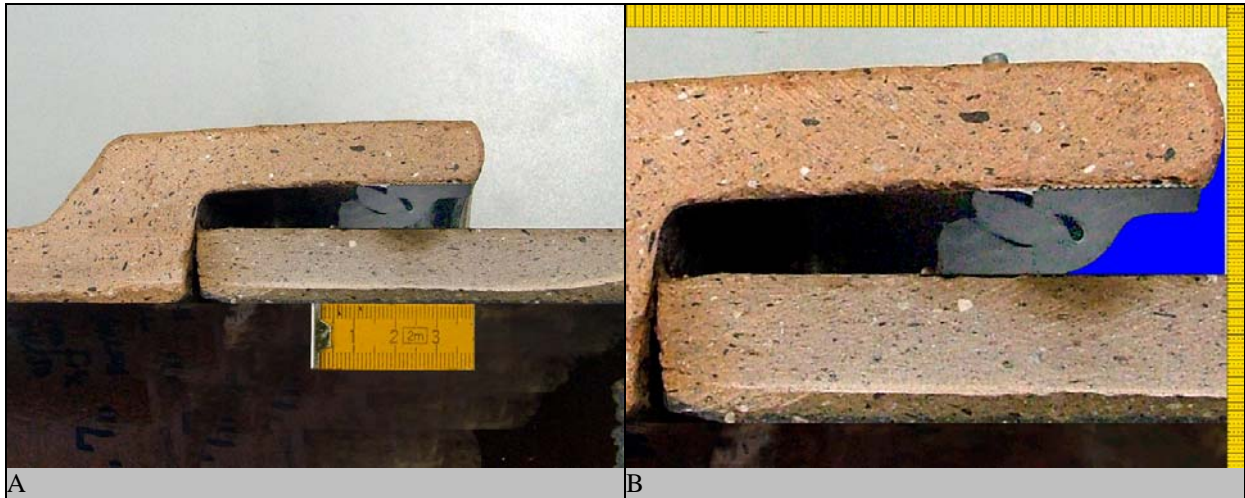
Abb. 102: Untersuchung der Verbindungsgeometrie. Rohrverbindung Steinzeug Cerafix DN 150. A Längsschnitt durch die Rohrverbindung. B Detail des Dichtelementes. Ringspalt = 7,0 mm. Der blau gekennzeichnete Raum vor dem Dichtelement hat im Längsschnitt eine Fläche von 117 mm 2 .
