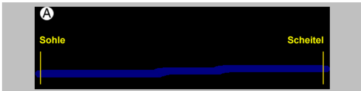
Abb. 22: Anpressdruckbild einer Rohrverbindung von der Rohrsohle bis zum Rohrscheitel ohne Scherlast.
