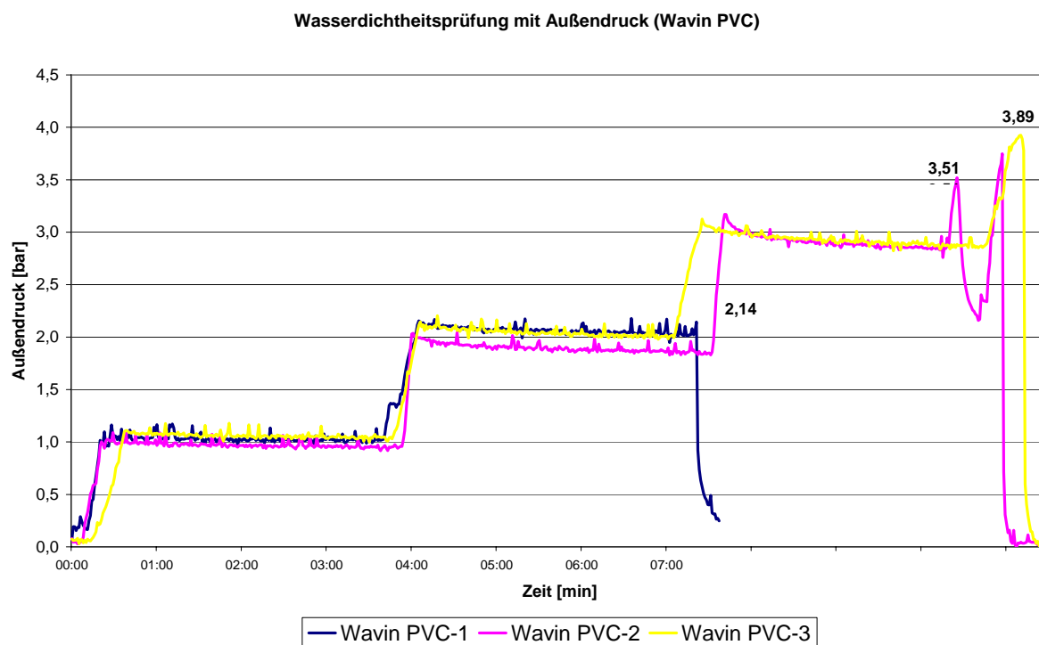
Abb. 65: Ergebnisse der Außendruckuntersuchungen an Rohrverbindungen vom Typ Wavin PVC-KG. Im Diagramm sind die Messwerte dreier Messungen aufgetragen. Die Höchstwerte geben den Versagensdruck bei den einzelnen Rohrverbindungen wieder.
