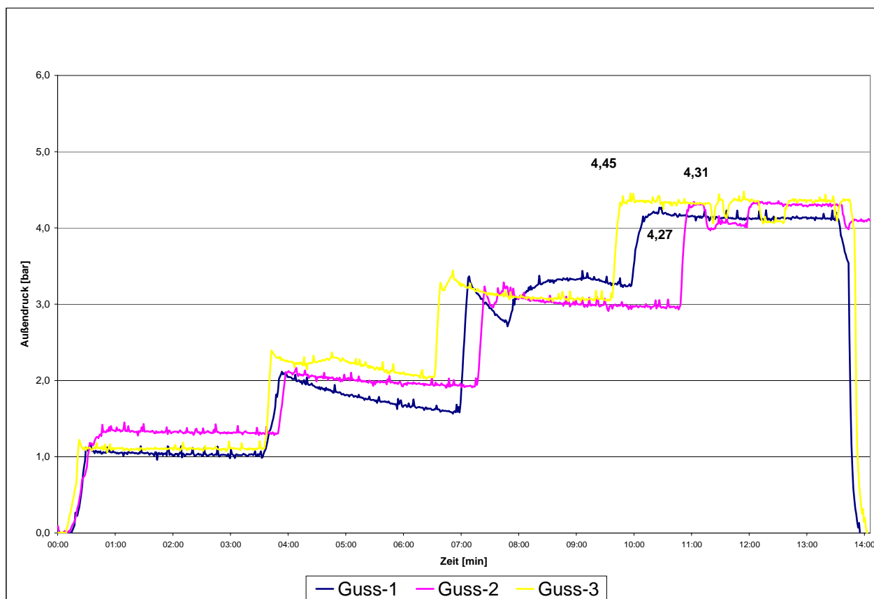
Abb. 90: Ergebnisse der Außendruckuntersuchungen an Rohrverbindungen vom Typ Integral Muffenrohr Standard, DN 150 der Saint-Gobain Gussrohr GmbH. Im Diagramm sind die Messwerte dreier Messungen aufgetragen. Die Höchstwerte geben den Höchstdruck des Wasserversorgungsnetzes wieder. Die sichtbaren Druckabfälle sind auf Undichtigkeiten im Versuchsstand zurückzuführen.
