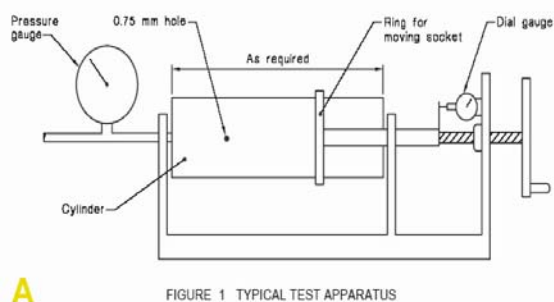
Abb. 15: Bestimmung des Anpressdrucks in der Rohrverbindung nach AS 1462 Part 13: A Schematische Darstellung des Versuchsaufbaus (vgl. [54]). B Versuchsstand mit Weg- und Druckmессeinrichtung (vgl. [54]).
