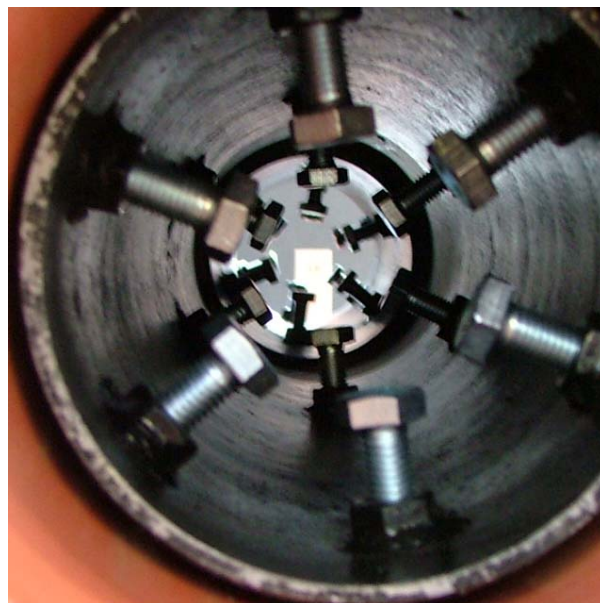
Abb.57: Rohrverbindung Awadukt SN4 PVC, bei einem Außenüberdruck von 2,0 bar. Kein Wassereintritt.
