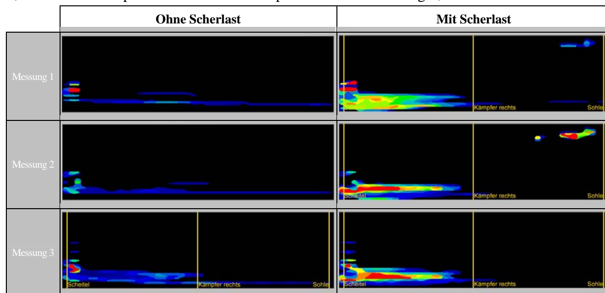
Abb. 26: Messung des Anpressdruckes mittels einer Druckfolie. Rohrverbindung Euroceramic Eurotrade DN 150 ohne Scherlast und mit Scherlast nach DIN [5]. Maßgeblicher Anpressdruck im Bereich der Rohrsohle: Messung 1) ohne Scherlast-Wirkung 2,3 bar, mit Scherlast-Wirkung 1,1 bar Messung 2) ohne Scherlast-Wirkung 1,1 bar, mit Scherlast-Wirkung 0,1 bar, Messung 3) ohne Scherlast-Wirkung 1,1 bar, mit Scherlast-Wirkung 0,1 bar. Mittelwerte des Anpressdruckes ohne Scherlast 1,5 bar , mit Scherlast 0,4 bar .
