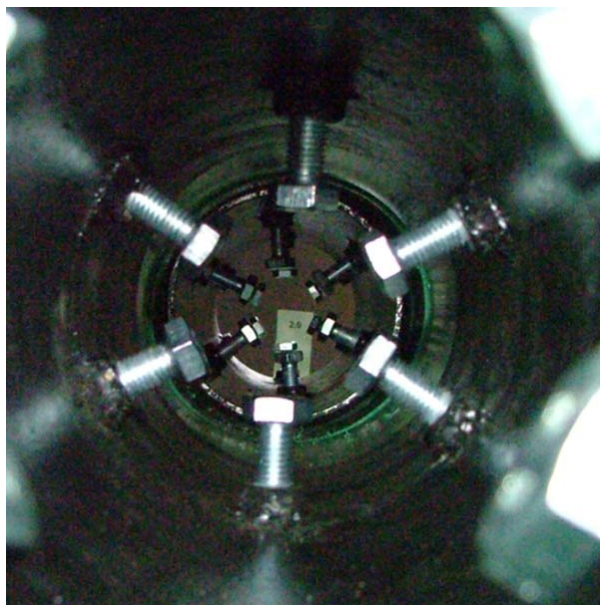
Abb.77: Rohrverbindung Rehau Awadukt PP SN 4 bei einem Außenüberdruck von 2,0 bar. Kein Wassereintritt.
