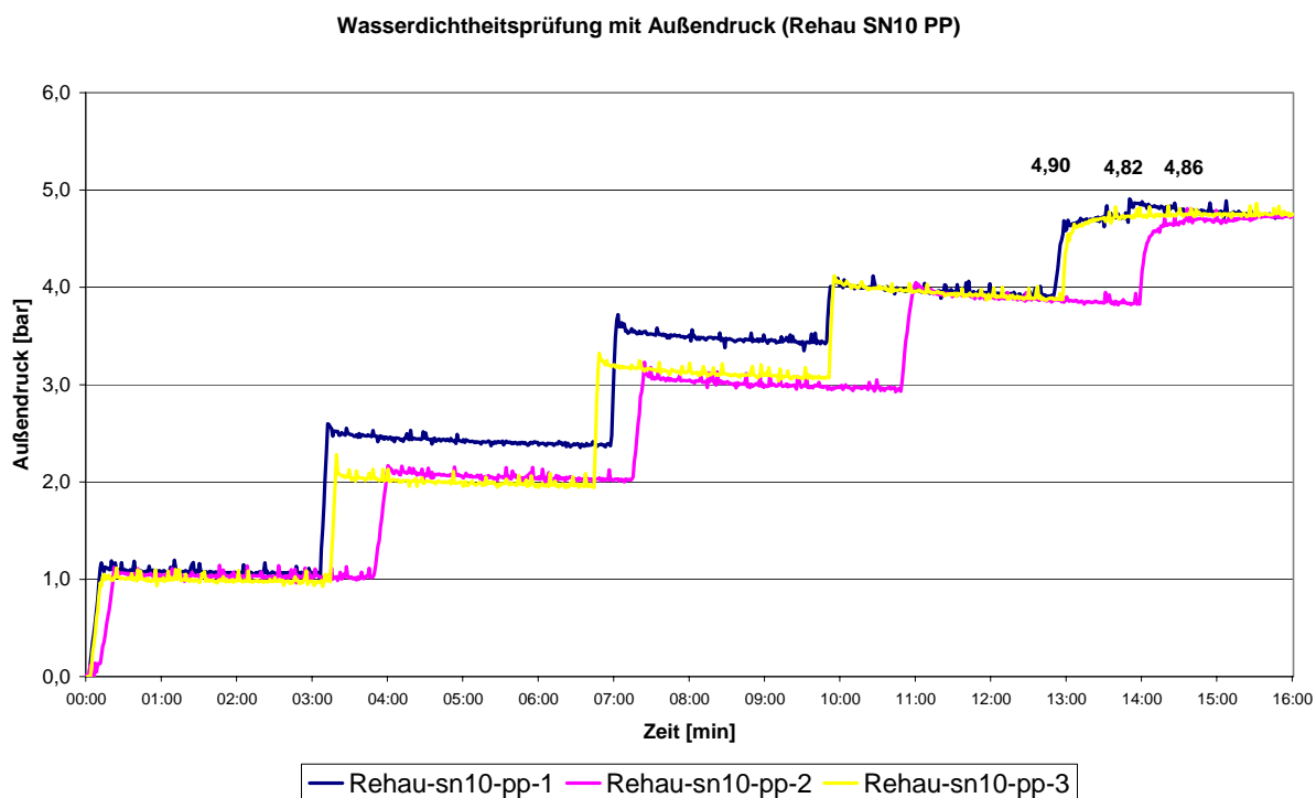
Abb. 85: Ergebnisse der Außendruckuntersuchungen an Rohrverbindungen vom Typ Rehau Awadukt SN 10 Rausisto. Im Diagramm sind die Messwerte dreier Messungen aufgetragen. Die Höchstwerte geben den Höchstdruck des Wasserversorgungsnetzes wieder.
