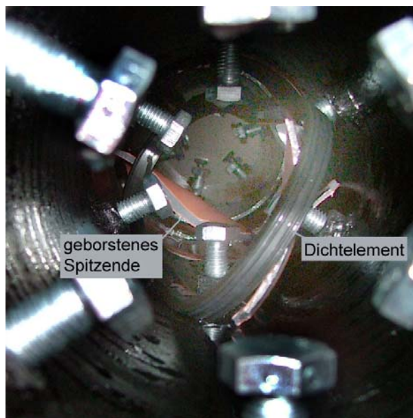
Abb.59: Rohrverbindung Awadukt SN4 PVC, nach einem maximalen Außenüberdruck von 4,03 bar. Wassereintritt durch Einbrechen des Spitzendes. Elastomerdichtung ist im Rohr erkennbar.
