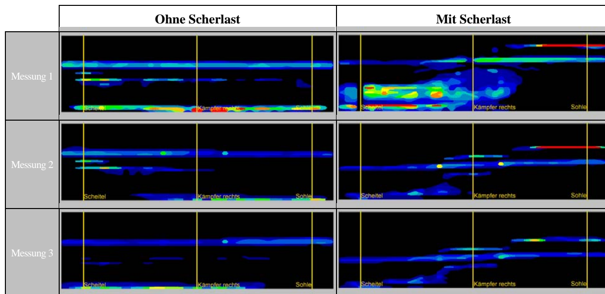
Abb. 34: Messung des Anpressdruckes mittels einer Druckfolie. Rohrverbindung Rehau Rausisto SN10 PP DN/OD 160 ohne Scherlast und mit Scherlast nach DIN [4]. Maßgeblicher Anpressdruck im Bereich der Rohrsohle: Messung 1) ohne Scherlast-Wirkung 9,1 bar, mit Scherlast-Wirkung 8,9 bar Messung 2) ohne Scherlast-Wirkung 3,7 bar, mit Scherlast-Wirkung 3,4 bar, Messung 3) ohne Scherlast-Wirkung 6,6 bar, mit Scherlast-Wirkung 6,5 bar. Mittelwerte des Anpressdruckes ohne Scherlast 6,5 bar , mit Scherlast 6,3 bar .
