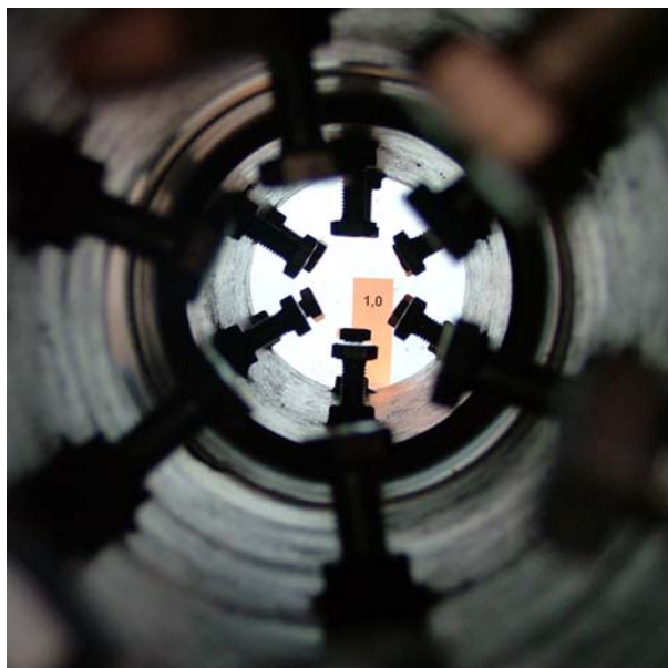
Abb.81: Rohrverbindung Rehau Awadukt SN 10 Rausisto, bei einem Außenüberdruck von 1,0 bar. Kein Wassereintritt.
