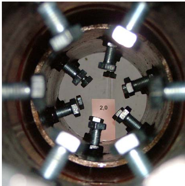
Abb.62: Rohrverbindung Wavin KG PVC bei einem Außenüberdruck von 2,0 bar. Kein Wassereintritt.
