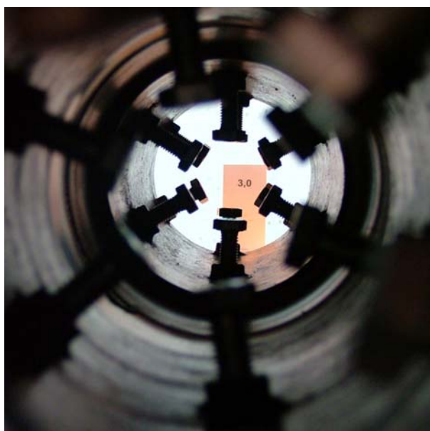
Abb.83: Rohrverbindung Rehau Awadukt SN 10 Rausisto, bei einem Außenüberdruck von 3,0 bar. Kein Wassereintritt.
