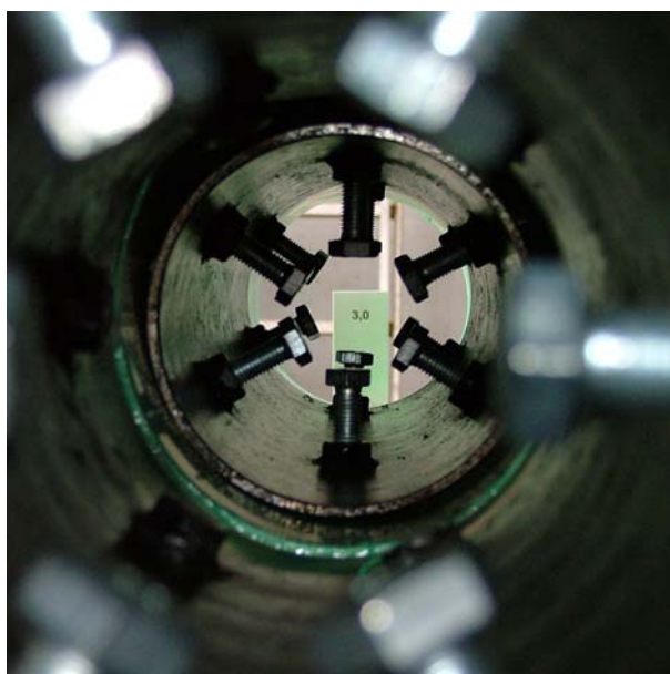
Abb.73: Rohrverbindung Ostendorf KG-2000 PP, bei einem Außenüberdruck von 3,0 bar. Kein Wassereintritt.
