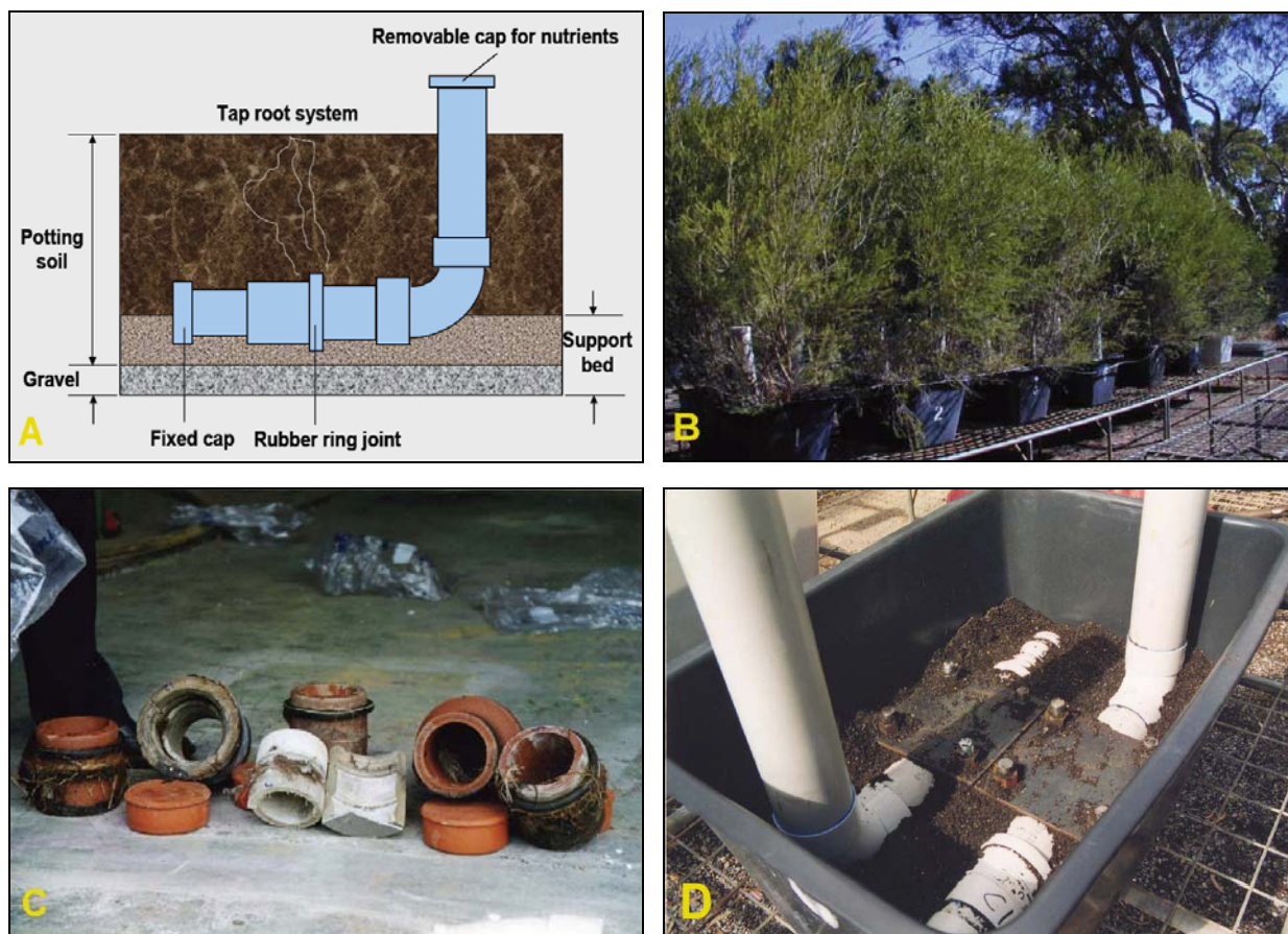
Abb. 17: Horizontal-Versuche des CSIRO, Australien: A Schematische Darstellung des Versuchsaufbaus. B Bepflanzte Versuchsgefäße. C Rohrverbindungen aus unterschiedlichen Werkstoffen nach dem Ausbau. D Verformung des Spitzendes mit Hilfe einer Stahlplatte.
