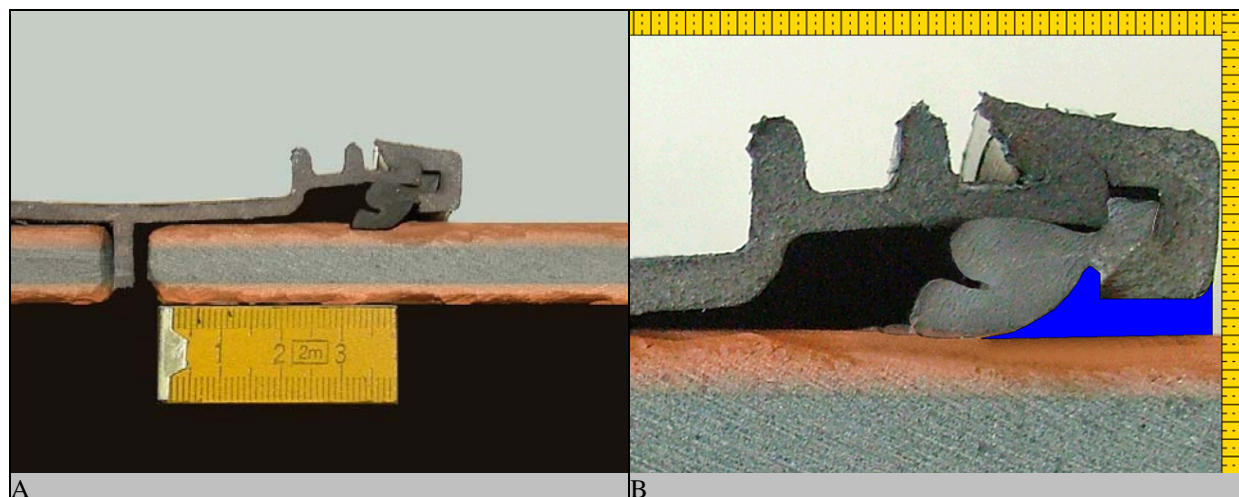
Abb. 104: Untersuchung der Verbindungsgeometrie. Rohrverbindung Euroceramic Eurotop, DN 150. A Längsschnitt durch die Rohrverbindung. B . Detail des Dichtelementes. Ringspalt = 3,7 mm. Der blau gekennzeichnete Raum vor dem Dichtelement hat im Längsschnitt eine Fläche von 26,34 mm 2 .
