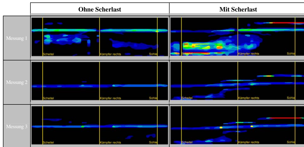
Abb. 30: Messung des Anpressdruckes mittels einer Druckfolie. Rohrverbindung Wavin KG PVC DN 150 ohne Scherlast und mit Scherlast nach DIN [4]. Maßgeblicher Anpressdruck im Bereich der Rohrsohle: Messung 1) ohne Scherlast-Wirkung 4,8 bar, mit Scherlast-Wirkung 3,9 bar Messung 2) ohne Scherlast-Wirkung 3,3 bar mit Scherlast-Wirkung 4,2 bar, Messung 3) ohne Scherlast-Wirkung 4,1 bar, mit Scherlast-Wirkung 3,0 bar. Mittelwerte des Anpressdruckes ohne Scherlast 4,1 bar , mit Scherlast 3,7 bar .
