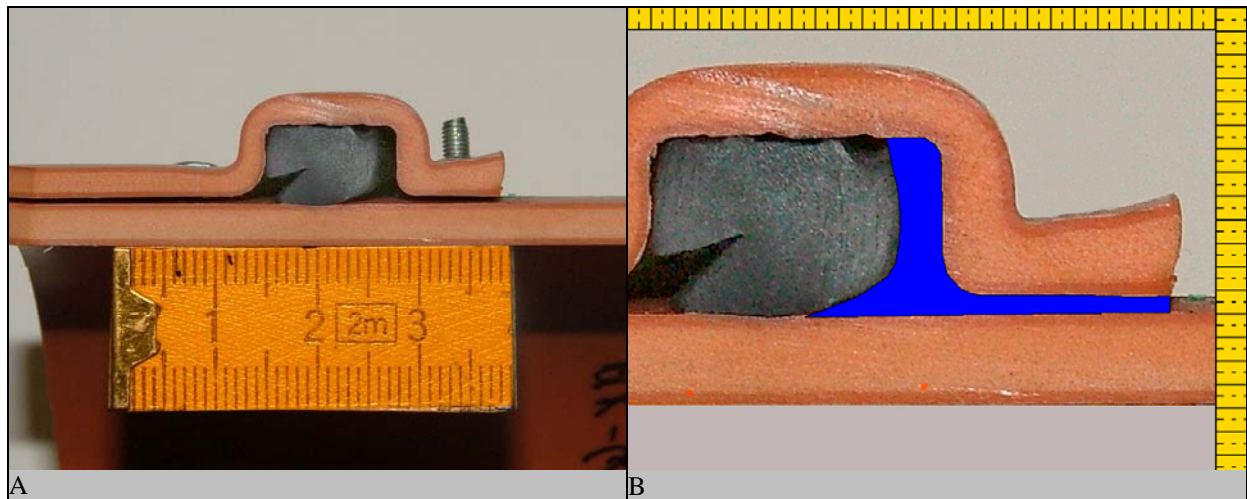
Abb. 107: Untersuchung der Verbindungsgeometrie. Rohrverbindung Wavin KG-PVC DN 150. A Längsschnitt durch die Rohrverbindung. B Detail des Dichtelementes. Ringspalt = 0,4 mm. Der blau gekennzeichnete Raum vor dem Dichtelement hat eine Fläche von 23 mm 2 .
