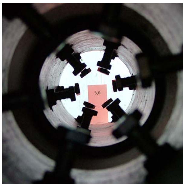
Abb.68: Rohrverbindung Awadukt PVC SN8, bei einem Außenüberdruck von 3,0 bar. Kein Wassereintritt.
