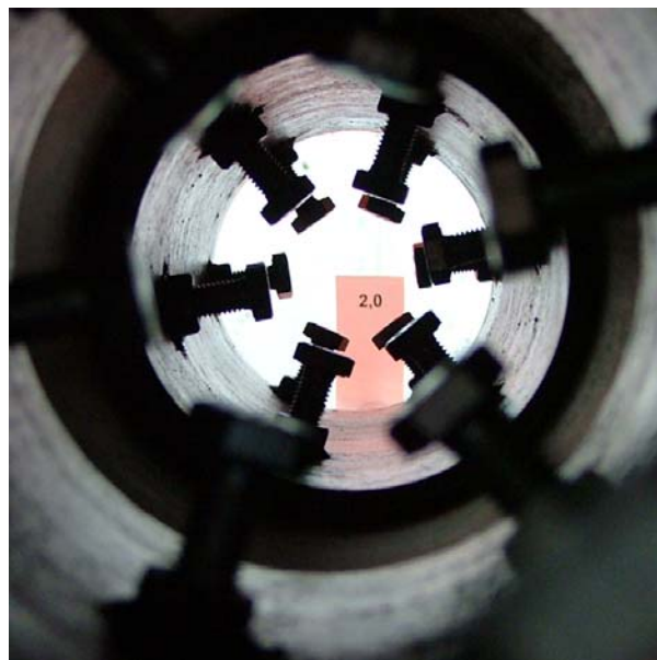
Abb.67: Rohrverbindung Awadukt PVC SN8, bei einem Außenüberdruck von 2,0 bar. Kein Wassereintritt.
