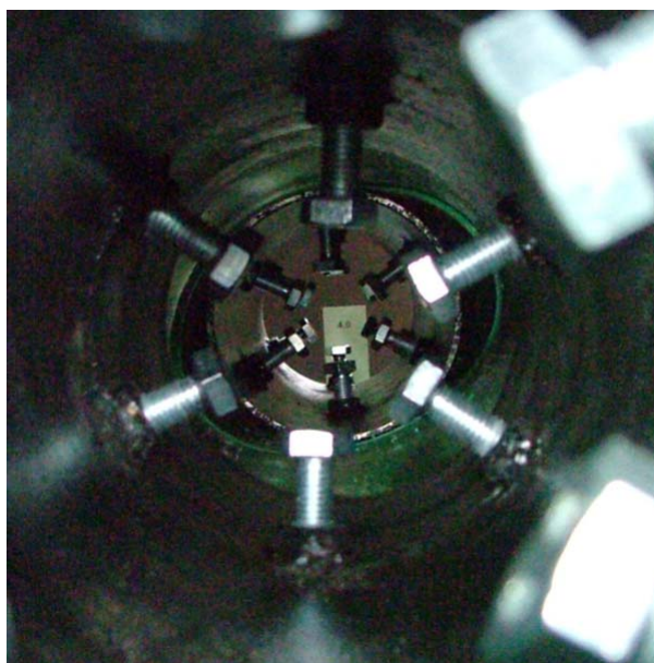
Abb.79: Rohrverbindung Rehau Awadukt PP SN 4 bei einem Außenüberdruck von 4,0 bar. Kein Wassereintritt trotz Beulen.
