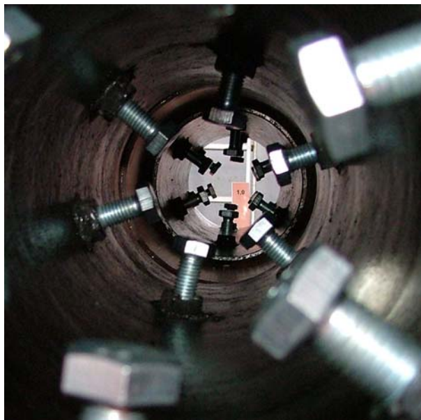
Abb.51: Rohrverbindung Ostendorf PVC-KG, bei einem Außenüberdruck von 1,0 bar. Kein Wassereintritt.
