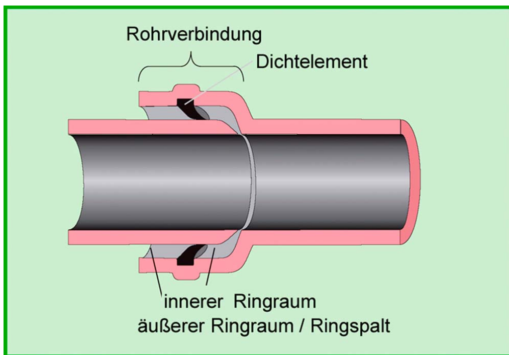
Abb. 18: Der äußere Ringraum einer Rohrverbindung ist für Wurzeln vom Bettungs- bzw. Verfüllmaterial aus erreichbar. Bei Durchwachsen des Dichtelementes erreichen sie den inneren Ringraum und damit den Leitungsquerschnitt.
