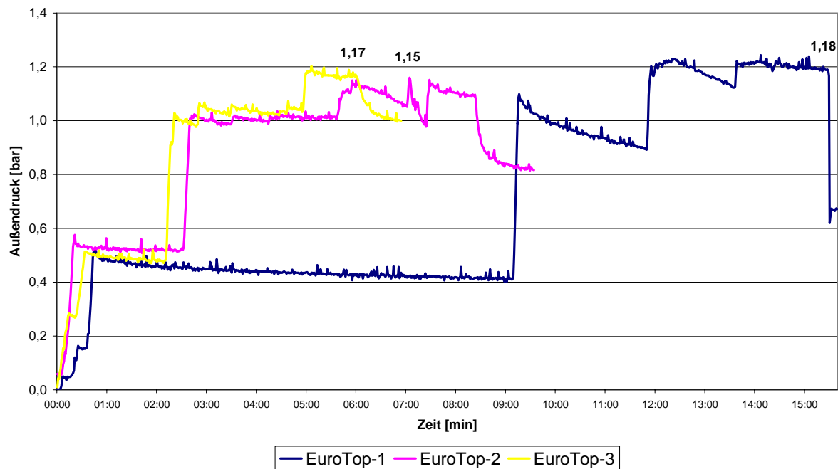
Abb. 50: Ergebnisse der Außenüberdruckuntersuchungen an Rohrverbindungen vom Typ Euroceramic Eurotop DN150. Im Diagramm sind die Messwerte dreier Messungen aufgetragen. Die Höchstwerte geben den Versagensdruck bei den einzelnen Rohrverbindungen wieder.
