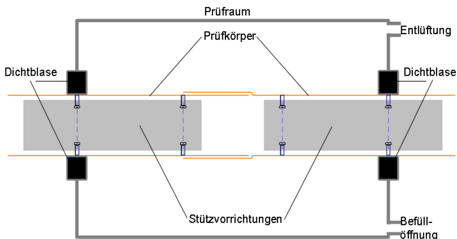
Abb. 38: Schema der Innendruckprüfanlage mit einem eingebauten Prüfkörper.
