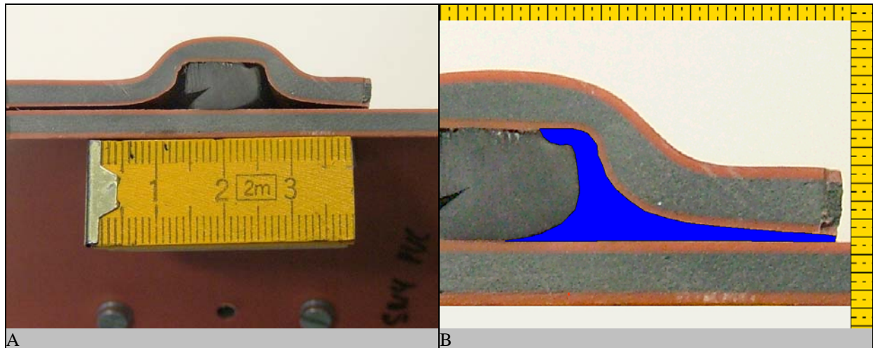
Abb. 106: Untersuchung der Verbindungsgeometrie. Rohrverbindung Awadukt SN4 PVC DN/OD 160. A Längsschnitt durch die Rohrverbindung. B Detail des Dichtelementes. Ringspalt = 0,3 mm. Der blau gekennzeichnete Raum vor dem Dichtelement hat eine Fläche von 33 mm 2 .
