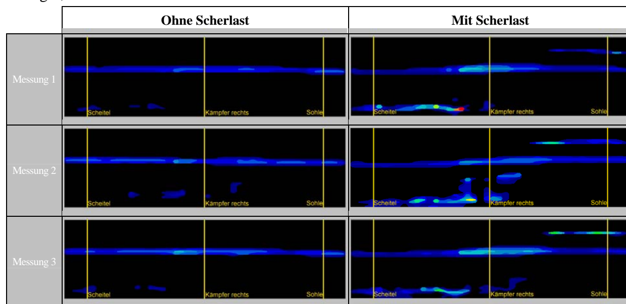
Abb. 33: Messung des Anpressdruckes mittels einer Druckfolie. Rohrverbindung Rehau Awadukt SN4 PP DN/OD 160 ohne Scherlast und mit Scherlast nach DIN [4]. Maßgeblicher Anpressdruck im Bereich der Rohrsohle: Messung 1) ohne Scherlast-Wirkung 4,8 bar, mit Scherlast-Wirkung 2,8 bar Messung 2) ohne Scherlast-Wirkung 4,1 bar, mit Scherlast-Wirkung 3,2 bar, Messung 3) ohne Scherlast-Wirkung 5,1 bar, mit Scherlast-Wirkung 3,6 bar. Mittelwerte des Anpressdruckes ohne Scherlast 4,7 bar , mit Scherlast 3,2 bar .
