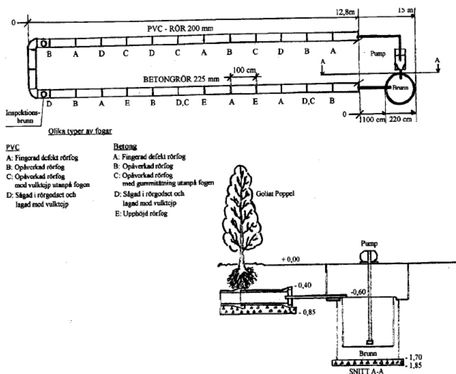
Abb. 11: Schema der Versuchsanlage in Schweden für Baumpflanzungen (Pappel) im Bereich von PVC- und Beton-Rohren (aus [48]).
