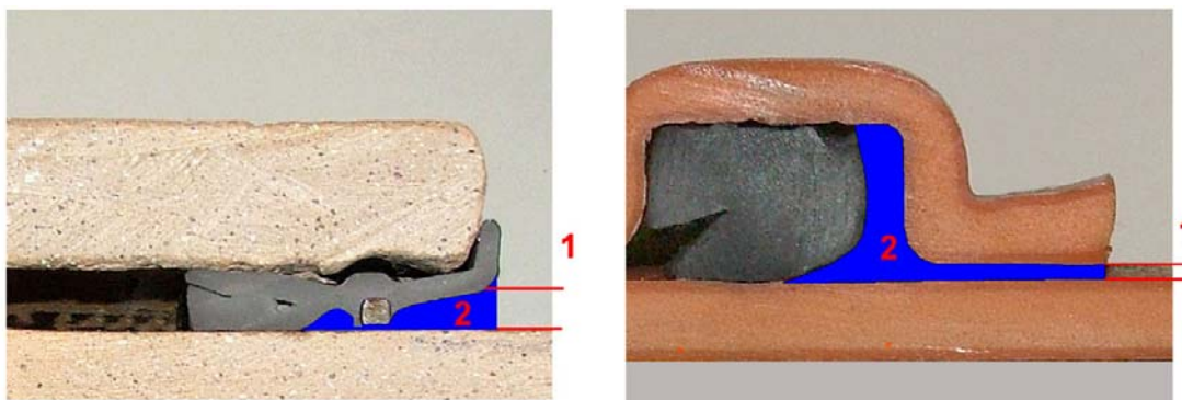
Abb. 101: Definition der Begriffe äußerer Ringspalt (1) und Ringraum (2) bei unterschiedlichen Verbindungstypen.
