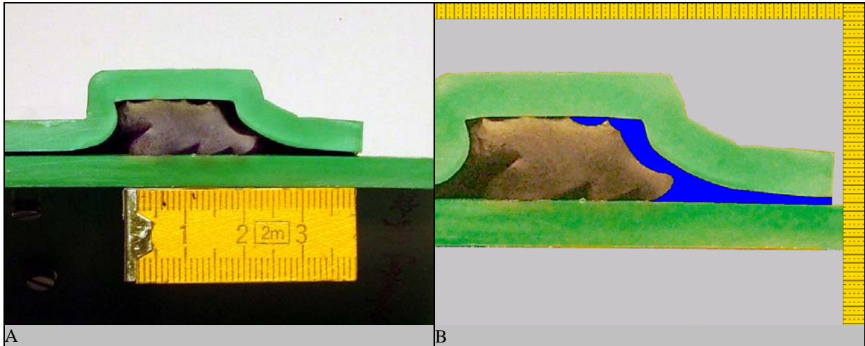
Abb. 109: Untersuchung der Verbindungsgeometrie. Rohrverbindung Ostendorf KG-2000 DN 150. A Längsschnitt durch die Rohrverbindung. B Detail Dichtelement. Ringspalt = 0,6 mm. Der blau gekennzeichnete Raum vor dem Dichtelement hat eine Fläche von 54 mm 2 .
