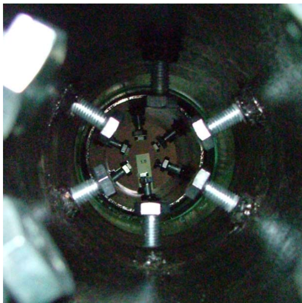
Abb.76: Rohrverbindung Rehau Awadukt SN PP 4 bei einem Außenüberdruck von 1,0 bar. Kein Wassereintritt.
