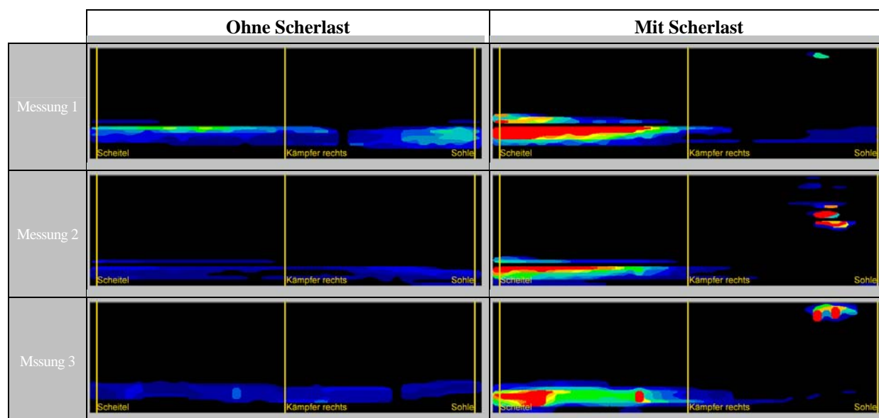
Abb. 25: Messung des Anpressdruckes mittels einer Druckfolie. Rohrverbindung Steinzeug Cerafix DN 150 ohne Scherlast und mit Scherlast nach DIN 4060 [4]. Maßgeblicher Anpressdruck im Bereich der Rohrsohle: Messung 1) ohne Scherlast-Wirkung 5,3 bar, mit Scherlast-Wirkung 0,4 bar Messung 2) ohne Scherlast-Wirkung 2,6 bar, mit Scherlast-Wirkung 0,1 bar, Messung 3) ohne Scherlast-Wirkung 1,0 bar, mit Scherlast-Wirkung 0,2 bar. Mittelwerte des Anpressdruckes ohne Scherlast 3,0 bar , mit Scherlast 0,2 bar .
