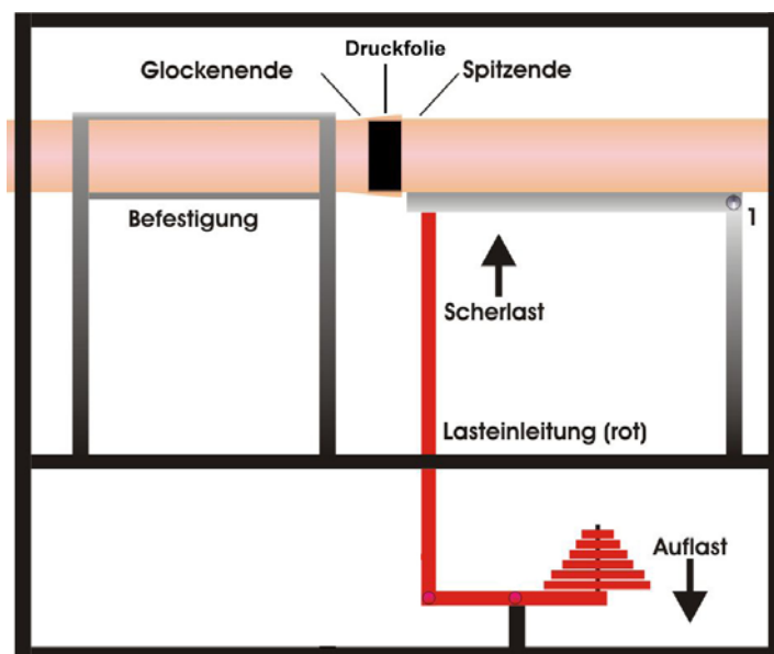
Abb. 19: Schematische Darstellung des Scherlastversuchs.
