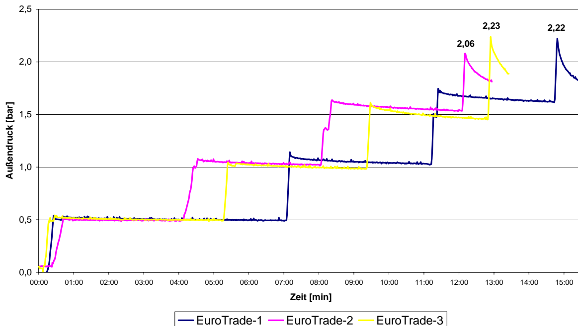
Abb. 47: Ergebnisse der Außendruckuntersuchungen an Rohrverbindungen vom Typ Euroceramic Eurotrade DN 150. Im Diagramm sind die Messwerte dreier Messungen aufgetragen. Die Höchstwerte geben den Versagensdruck bei den einzelnen Rohrverbindungen wieder.
