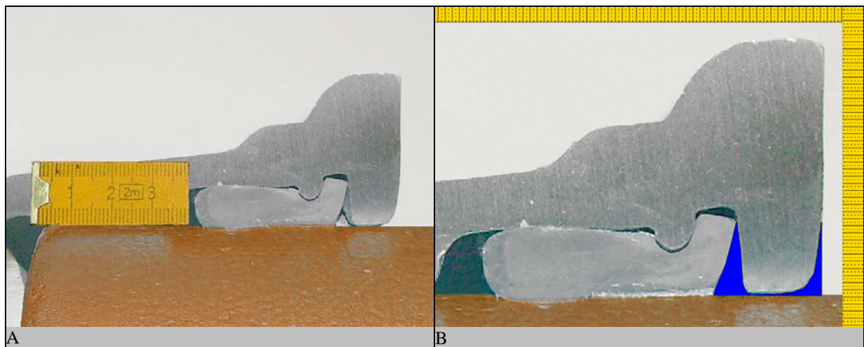
Abb. 112: Untersuchung der Verbindungsgeometrie. Rohrverbindung Gussrohr Tyton, DN 150. A Längsschnitt durch die Rohrverbindung. B Detail Dichtelement. Ringspalt = 0,8 mm. Der blau gekennzeichnete Raum vor dem Dichtelement hat eine Fläche von 37 mm 2 .
