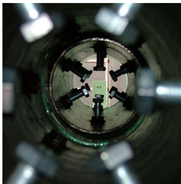
Abb.74: Rohrverbindung Ostendorf KG-2000 PP, bei einem Außenüberdruck von 4,0 bar. Kein Wassereintritt.
