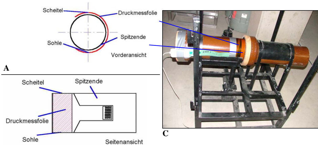
Abb. 21: Messung des Anpressdruckes bei Einwirken einer Scherlast. A Druckfolie auf dem Spitzende einer Rohrverbindung, Querschnitt. B Druckfolie auf dem Spitzende einer Rohrverbindung, Ansicht. C In den Scherlastversuchsstand eingebaute Rohrverbindung aus Keramik.
