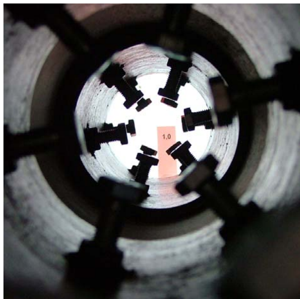
Abb.66: Rohrverbindung Awadukt PVC SN8, bei einem Außenüberdruck von 1,0 bar. Kein Wassereintritt.
