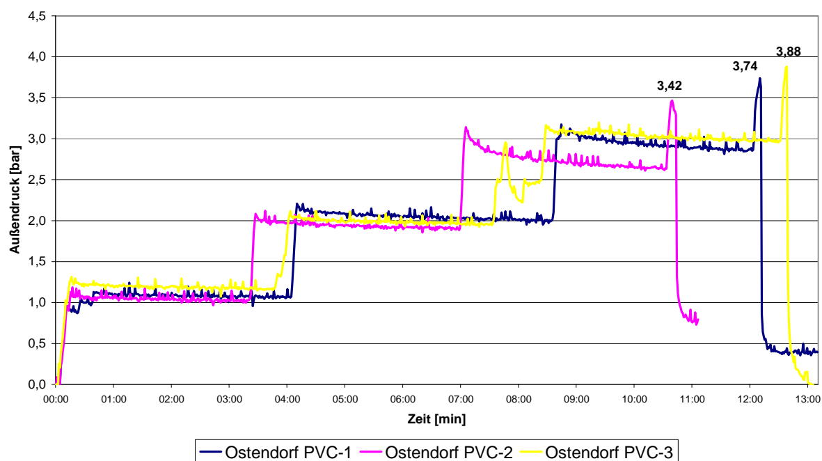
Abb. 55: Ergebnisse der Außendruckuntersuchungen an Rohrverbindungen vom Typ Ostendorf PVC-KG. Im Diagramm sind die Messwerte dreier Messungen aufgetragen. Die Druckmesswerte geben den Versagensdruck bei den einzelnen Rohrverbindungen wieder.
