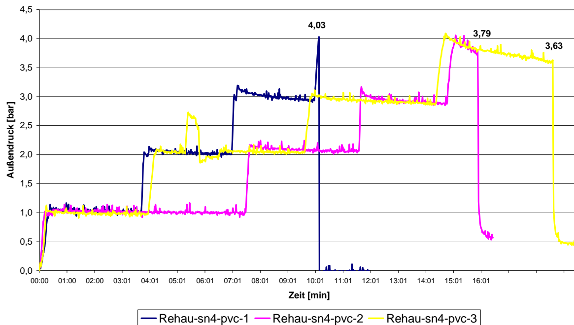
Abb. 60: Ergebnisse der Außenüberdruckuntersuchungen an Rohrverbindungen vom Typ Rehau PVC-SN4. Im Diagramm sind die Messwerte dreier Messungen aufgetragen. Die Höchstwerte geben den Versagensdruck bei den einzelnen Rohrverbindungen wieder.
