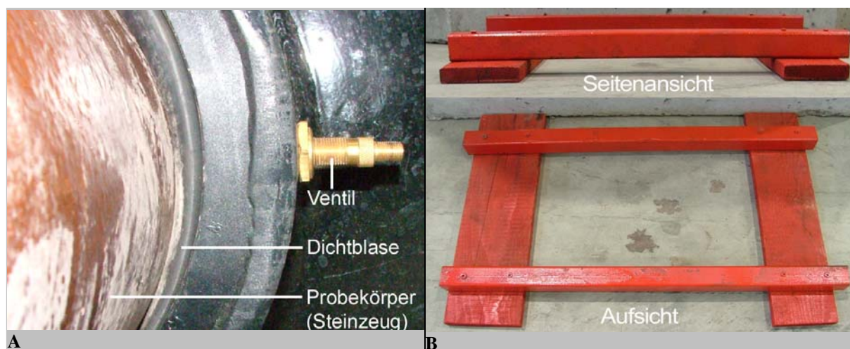
Abb. 40: Details der Vorrichtung zur Wasseraußendruckuntersuchung. A Der Abschluss des Prüfraumes erfolgt durch zwei Absperrblasen, welche die Außenoberfläche der Untersuchungsobjekte absperren. B Innerhalb der Vorrichtung befindet sich ein Auflager, mit dessen Hilfe die zu untersuchenden Rohrverbindungen horizontal ausgerichtet werden.
