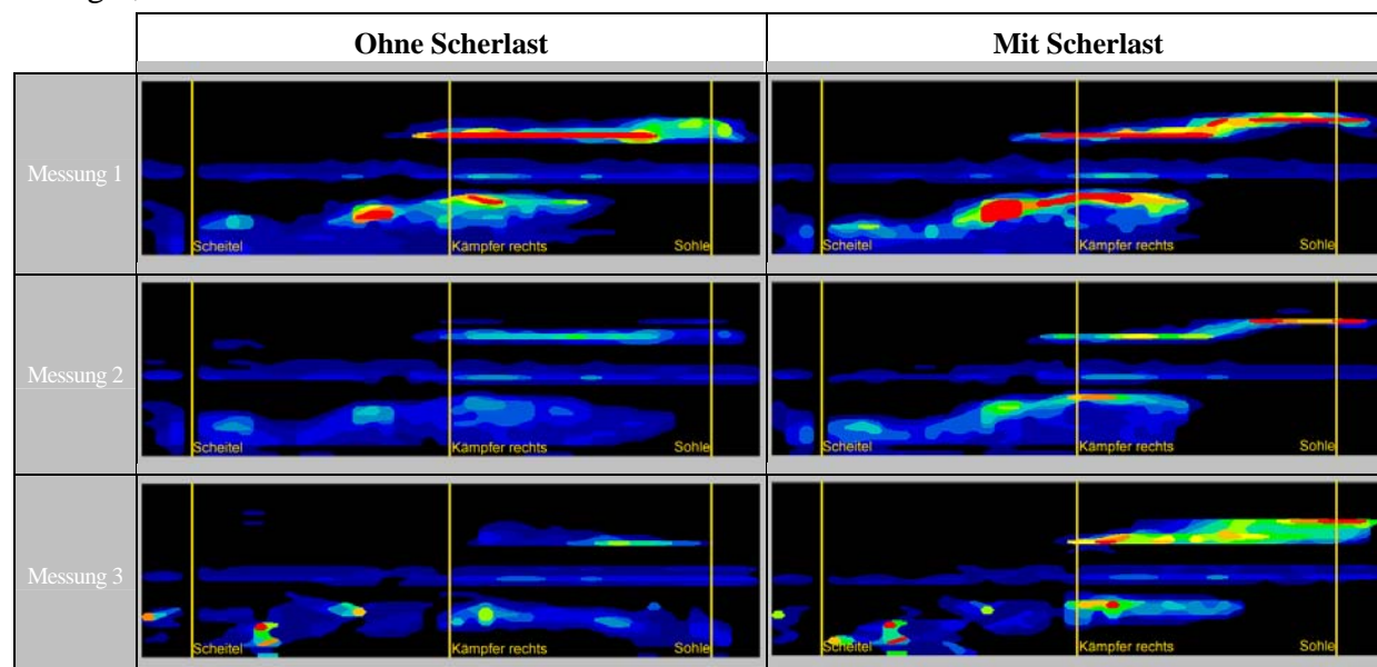
Abb. 31: Messung des Anpressdruckes mittels einer Druckfolie. Rohrverbindung Rehau Awadukt PVC SN8 DN/OD 160 ohne Scherlast und mit Scherlast nach DIN [4]. Maßgeblicher Anpressdruck im Bereich der Rohrsohle: Messung 1) ohne Scherlast-Wirkung 5,4 bar, mit Scherlast-Wirkung 2,0 bar Messung 2) ohne Scherlast-Wirkung 3,1 bar, mit Scherlast-Wirkung 1,3 bar, Messung 3) ohne Scherlast-Wirkung 2,8 bar mit Scherlast-Wirkung 1,7 bar. Mittelwerte des Anpressdruckes ohne Scherlast 3,8 bar , mit Scherlast 1,7 bar .
