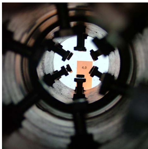
Abb.84: Rohrverbindung Rehau Awadukt SN 10 Rausisto, bei einem Außenüberdruck von 4,0 bar. Kein Wassereintritt.
