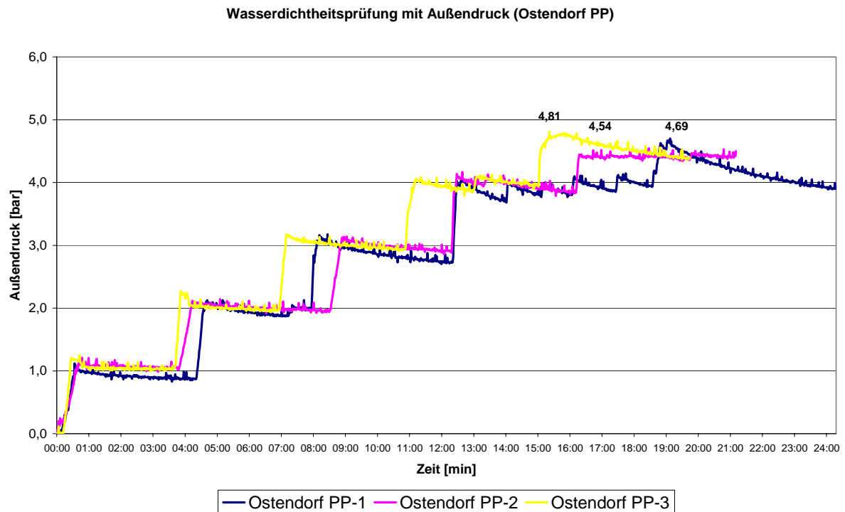
Abb. 75: Ergebnisse der Außendruckuntersuchungen an Rohrverbindungen vom Typ Ostendorf KG-2000 PP. Im Diagramm sind die Messwerte dreier Messungen aufgetragen. Die Höchstwerte geben den Höchstdruck des Wasserversorgungsnetzes wieder.
