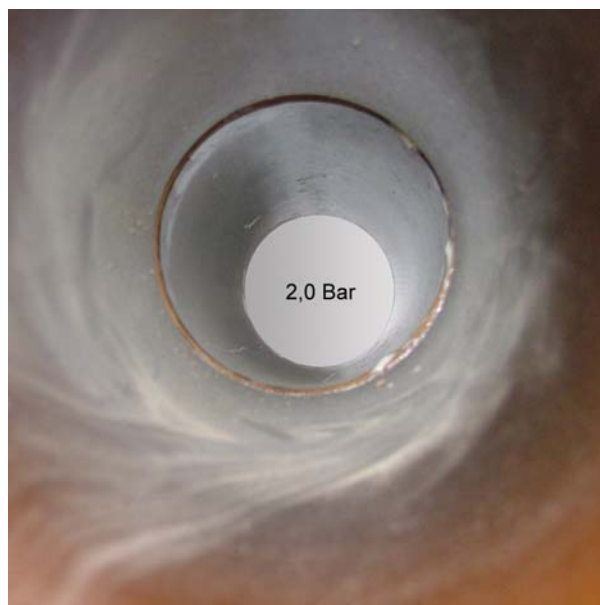
Abb.45: Rohrverbindung Euroceramic Eurotrade DN 150, bei einem Außenüberdruck von 2,0 bar. Kein Wassereintritt.
