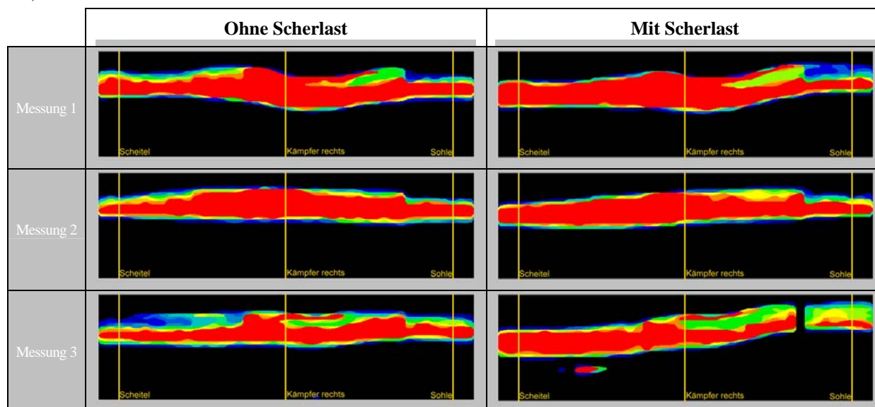
Abb. 35: Messung des Anpressdruckes mittels einer Druckfolie. Rohrverbindung Saint Gobain Gussrohr Tyton® DN 160 ohne Scherlast und mit Scherlast nach DIN [4]. Maßgeblicher Anpressdruck im Bereich der Rohrsohle: Messung 1) ohne Scherlast-Wirkung 24,8 bar, mit Scherlast-Wirkung 21,2 bar Messung 2) ohne Scherlast-Wirkung 23,9 bar, mit Scherlast 20,4 bar, Messung 3) ohne Scherlast-Wirkung 17,8 bar, mit Scherlast-Wirkung 10,8 bar. Mittelwerte des Anpressdruckes ohne Scherlast 22,2 bar , mit Scherlast 17,5 bar .
