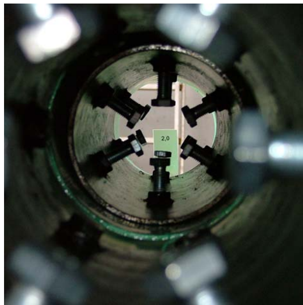
Abb.72: Rohrverbindung Ostendorf KG-2000 PP, bei einem Außenüberdruck von 2,0 bar. Kein Wassereintritt.
