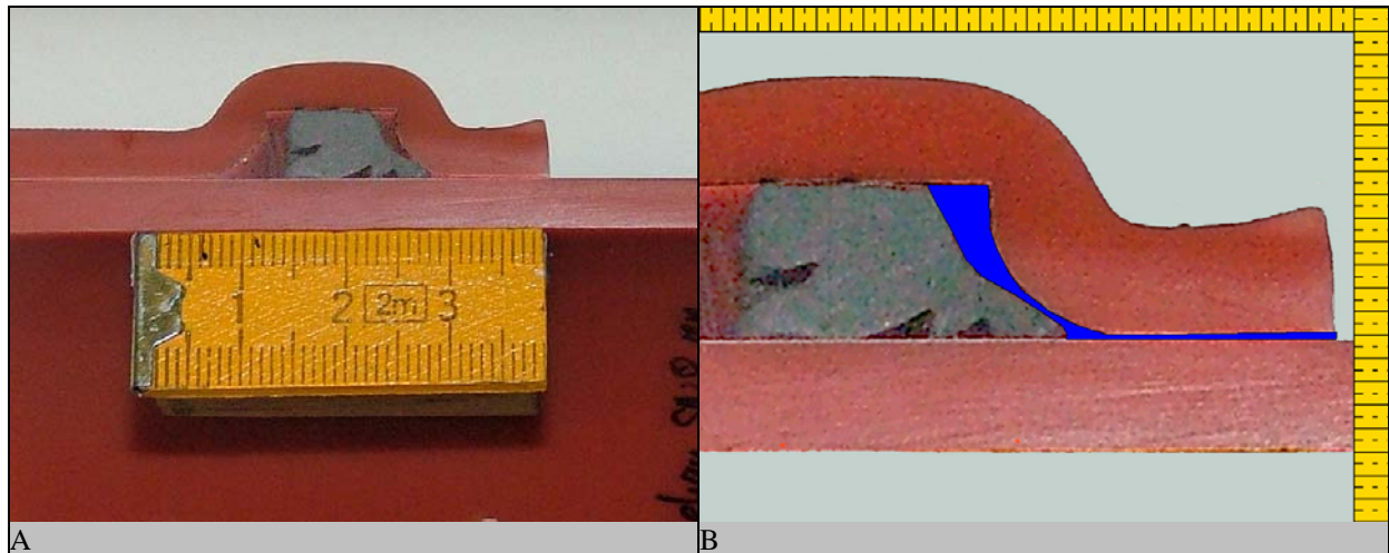
Abb. 108: Untersuchung der Verbindungsgeometrie. Rohrverbindung Rehau Awadukt PVC SN8 DN/OD 160. A Längsschnitt durch die Rohrverbindung. B Detail des Dichtelementes. Ringspalt = 0,3 mm. Der blau gekennzeichnete Raum vor dem Dichtelement hat eine Fläche von 12 mm 2 .
