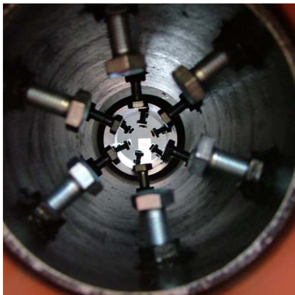
Abb.56: Rohrverbindung Awadukt SN4 PVC, bei einem Außenüberdruck von 1,0 bar. Kein Wassereintritt.
