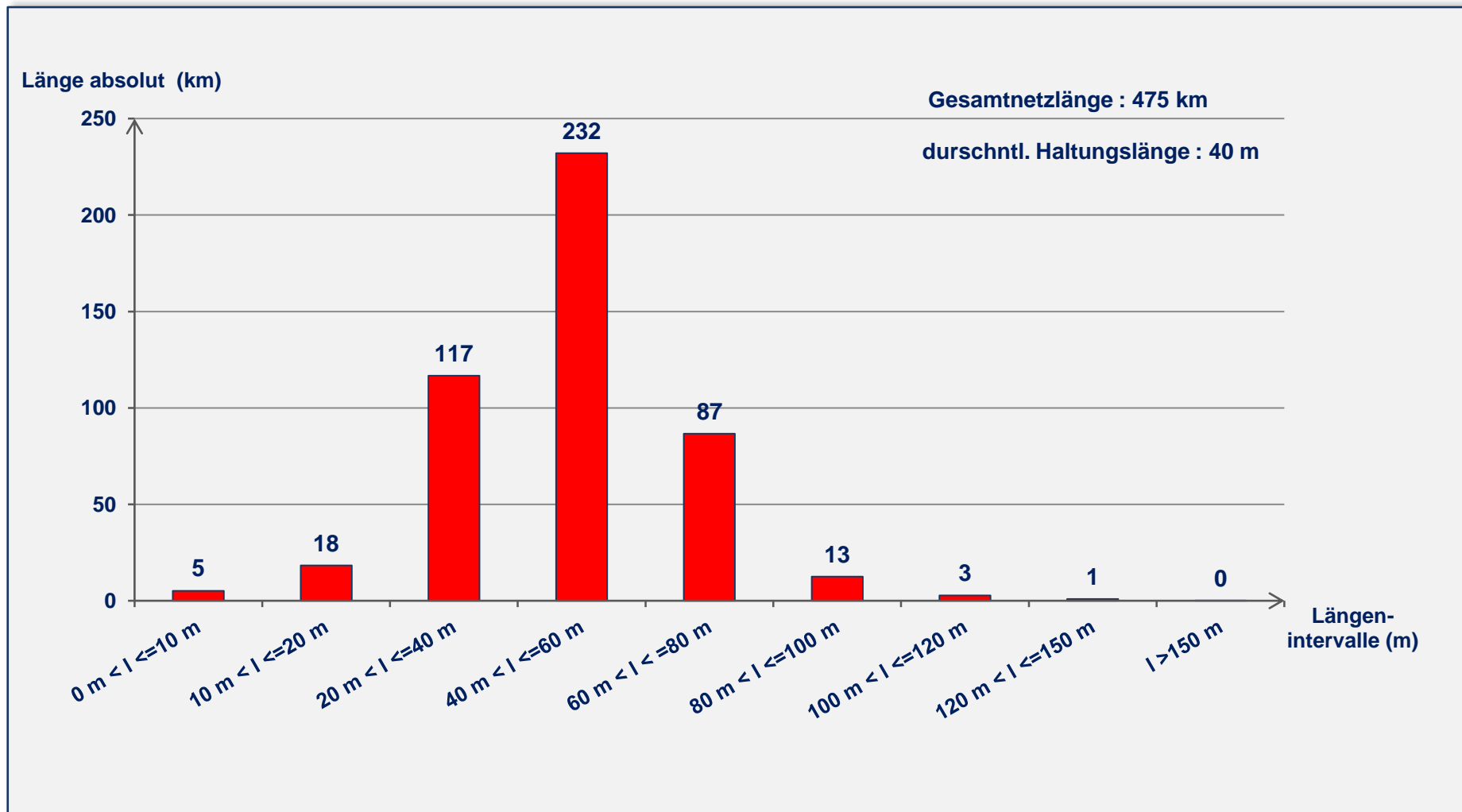
Abbildung A-1: Längenverteilung der Haltungen
