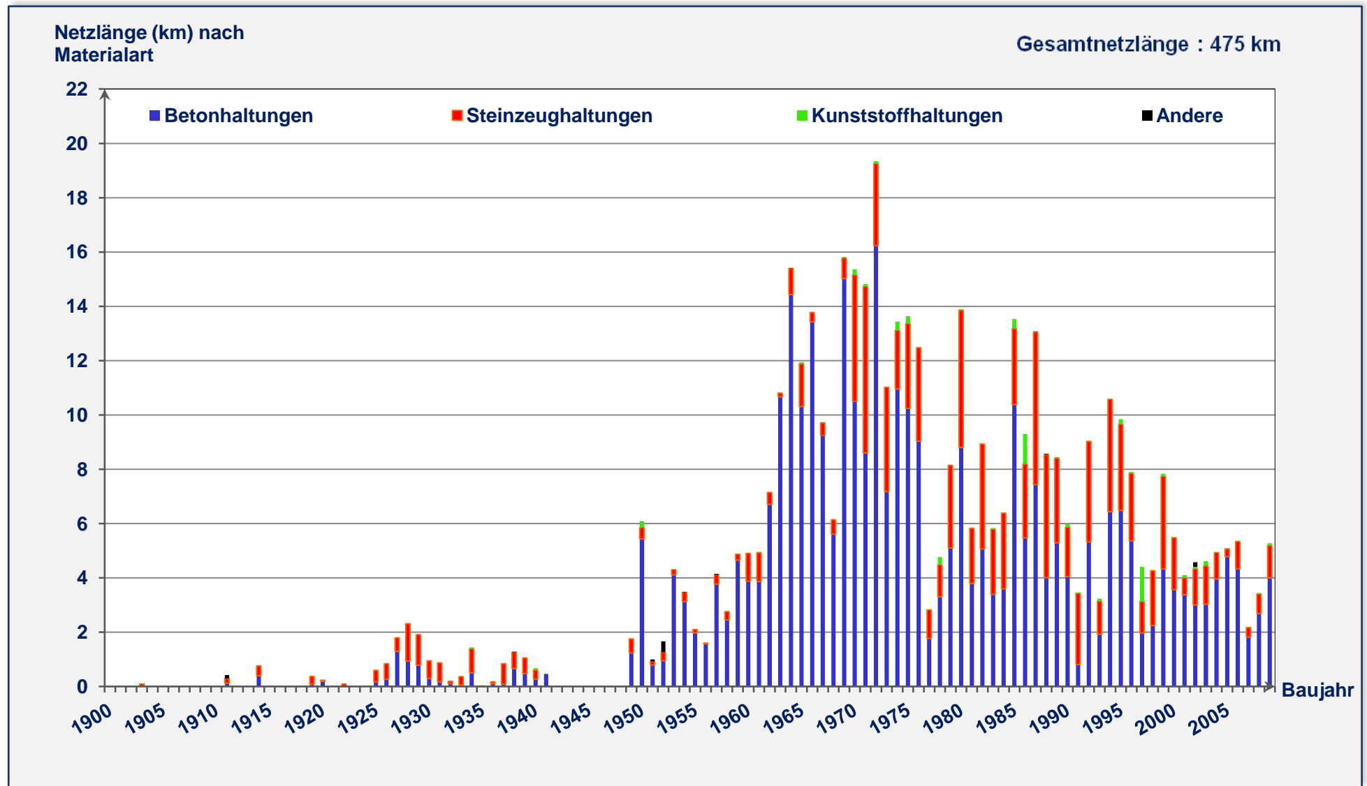
Abbildung A-2: Materialverteilung über Netzlänge und Baujahre in Rheine
