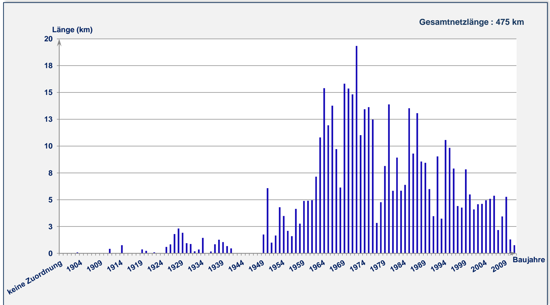
Abbildung A-3: Kanalnetzentwicklung in Rheine über Baujahre
