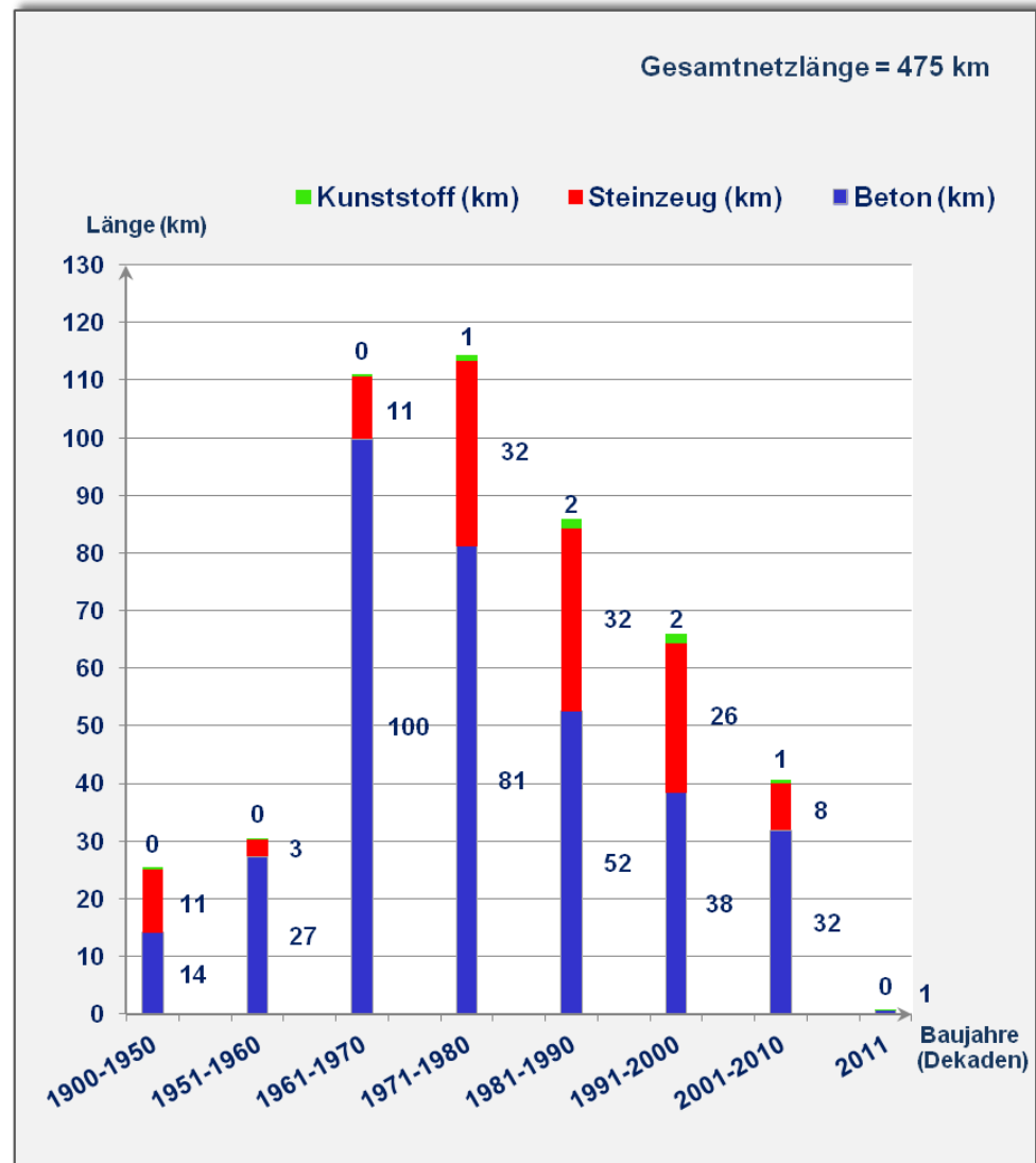
Abbildung A-7: Baustoffverteilung über Haltungen Rheine nach Dekaden
