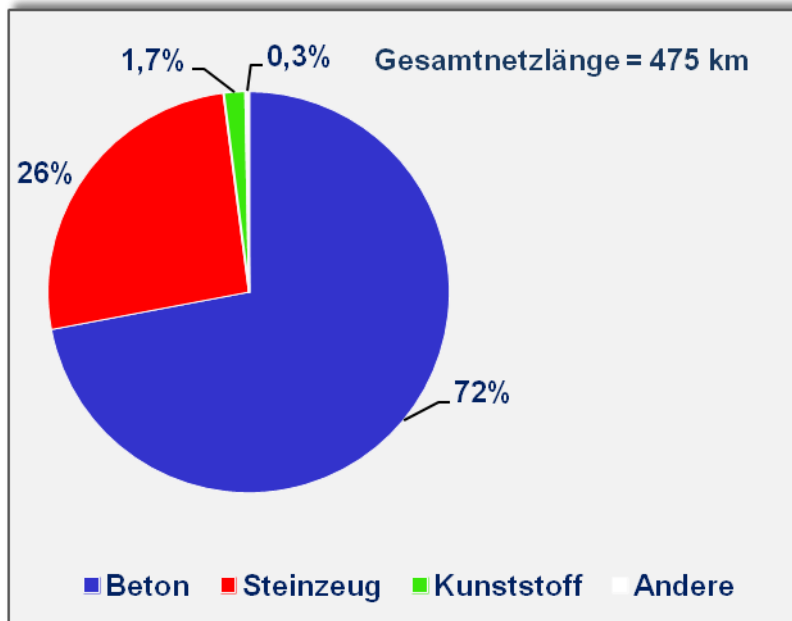
Abbildung A-6: Baustoffverteilung über Haltungen Rheine
