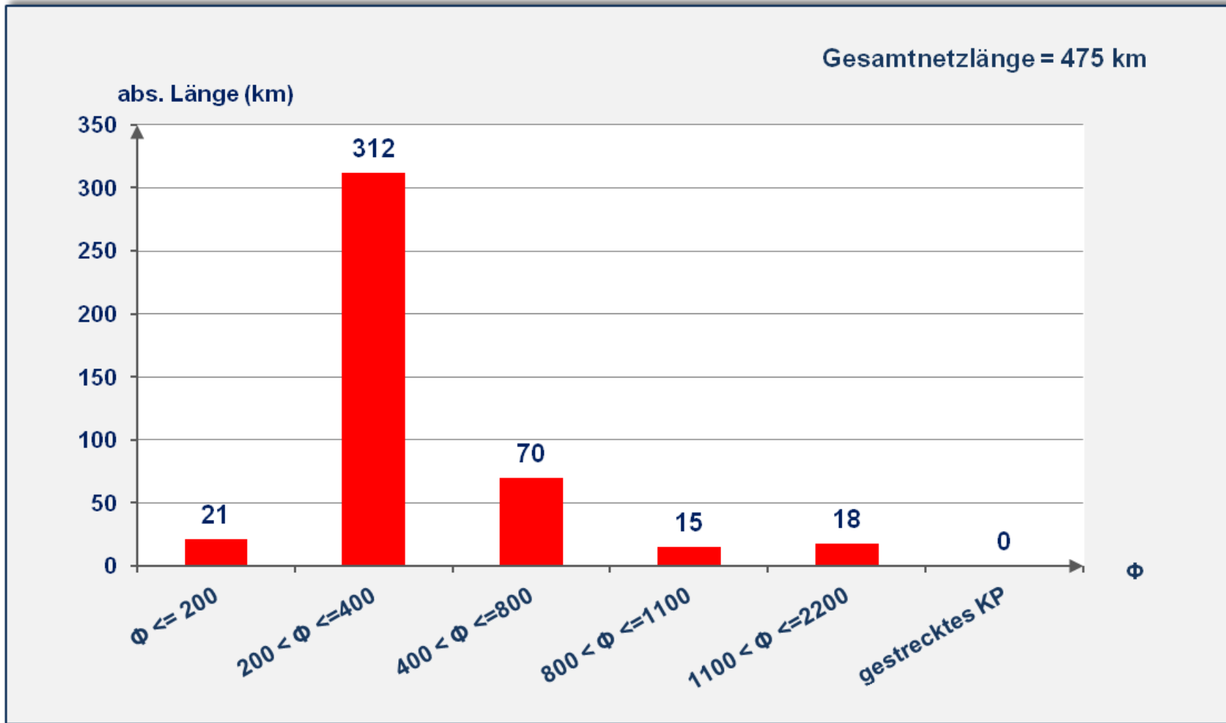
Abbildung A-5: Kreisprofilverteilung in Rheine über Länge
