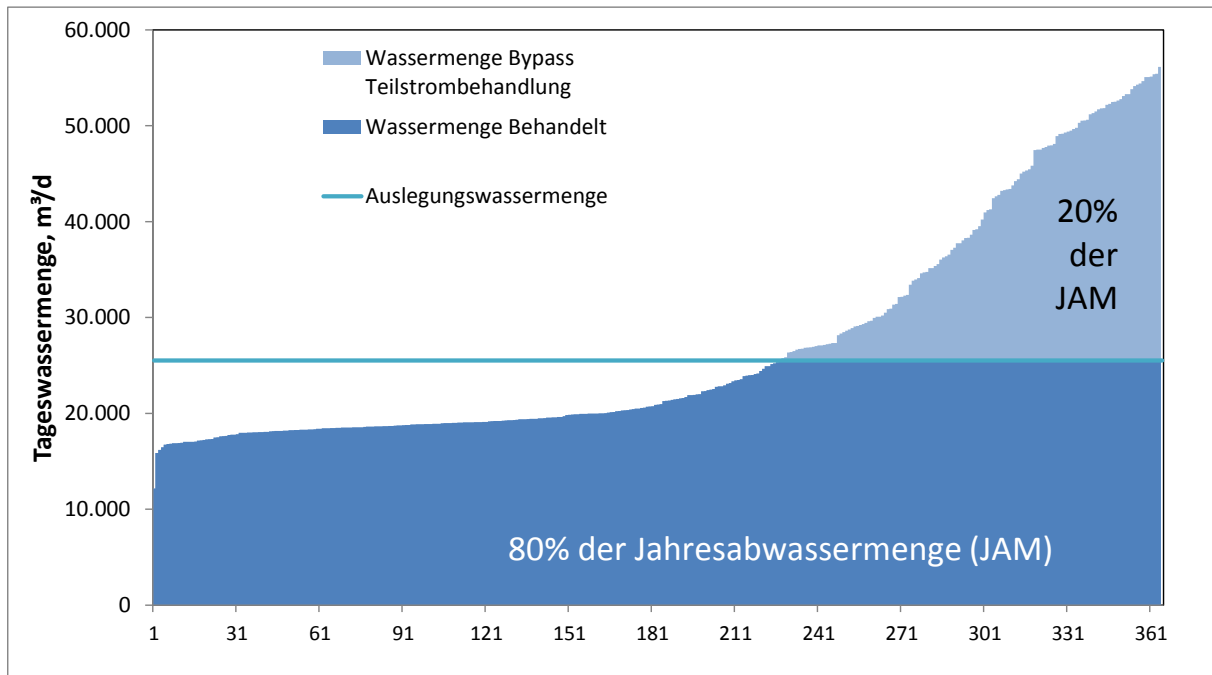
Abbildung 45: Behandelte Wassermenge und Bypassmenge bei der Teilstrombehandlung
