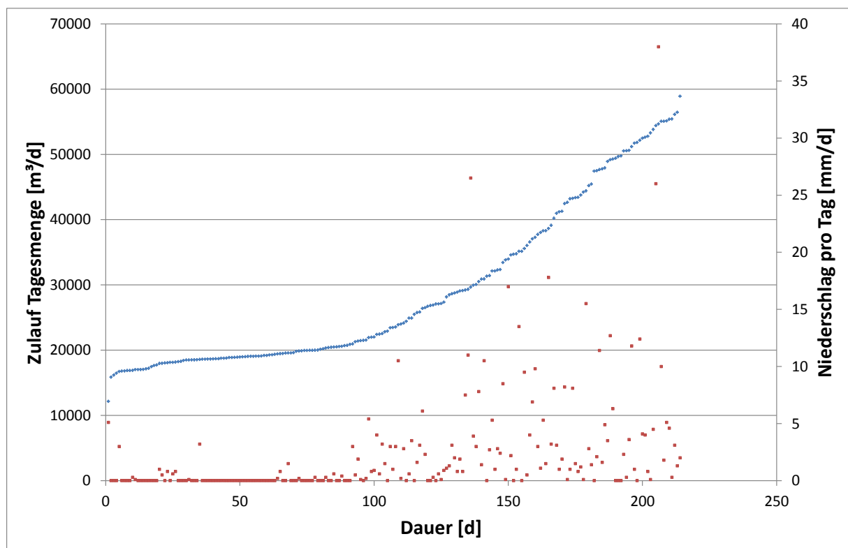
Abbildung 30: Häufigkeitsverteilung der Tageszuflüsse für das Jahr 2015, GWK Kenten
