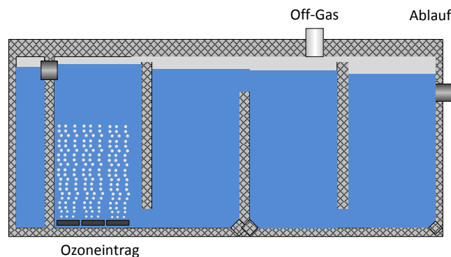
Abbildung 42: Prinzipskizze Ozon-Kontaktreaktor
