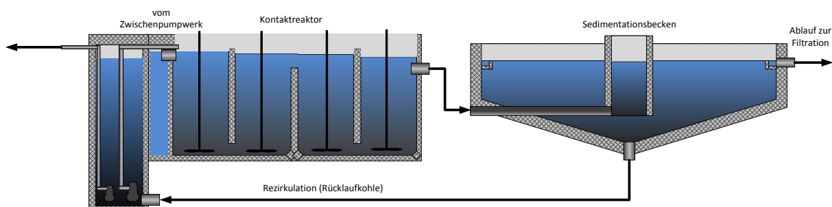
Abbildung 36: Systemskizze PAK-Stufe
