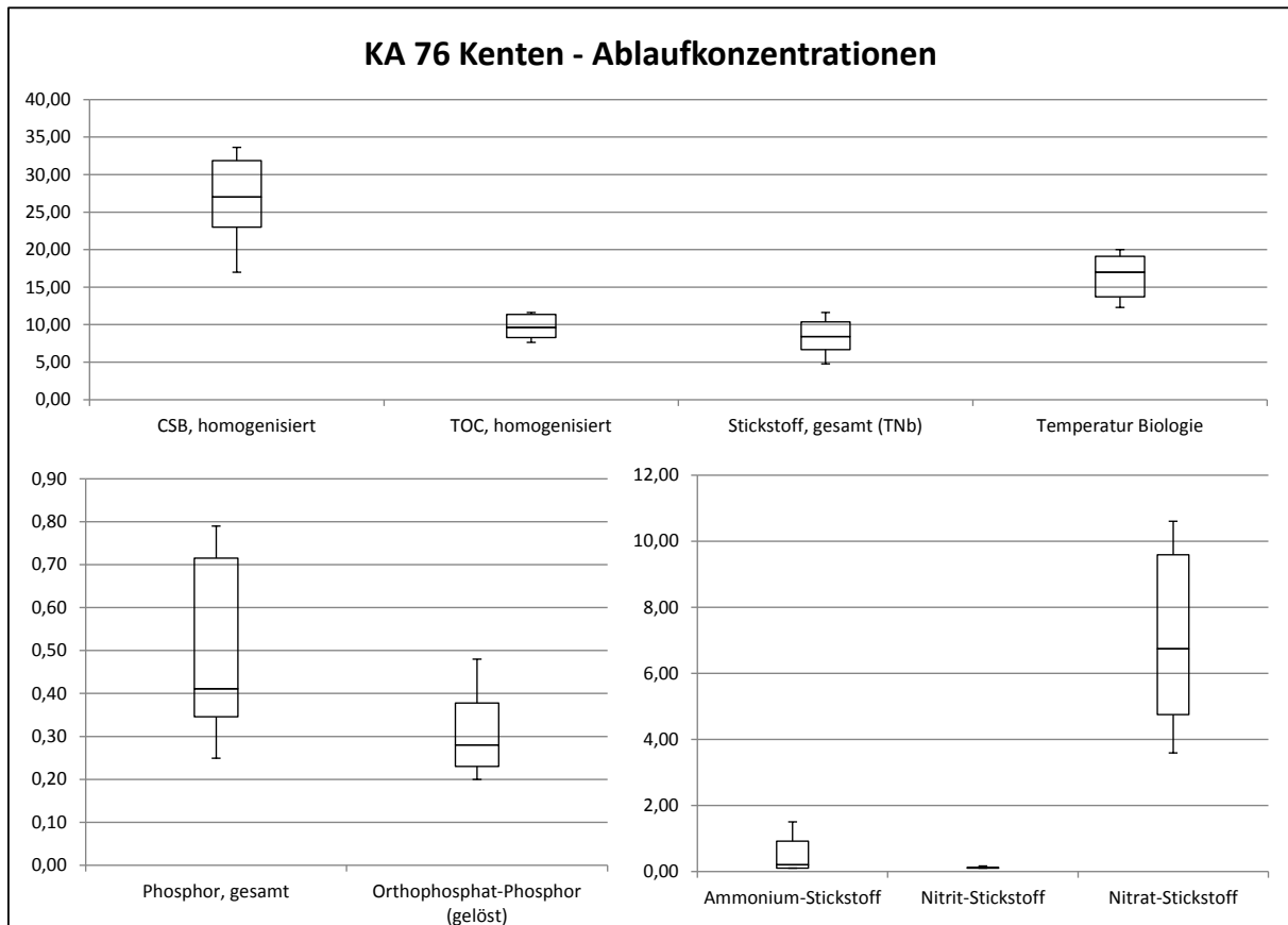
Abbildung 31: Ablaufkonzentrationen der Standardparameter GWK Kenten
