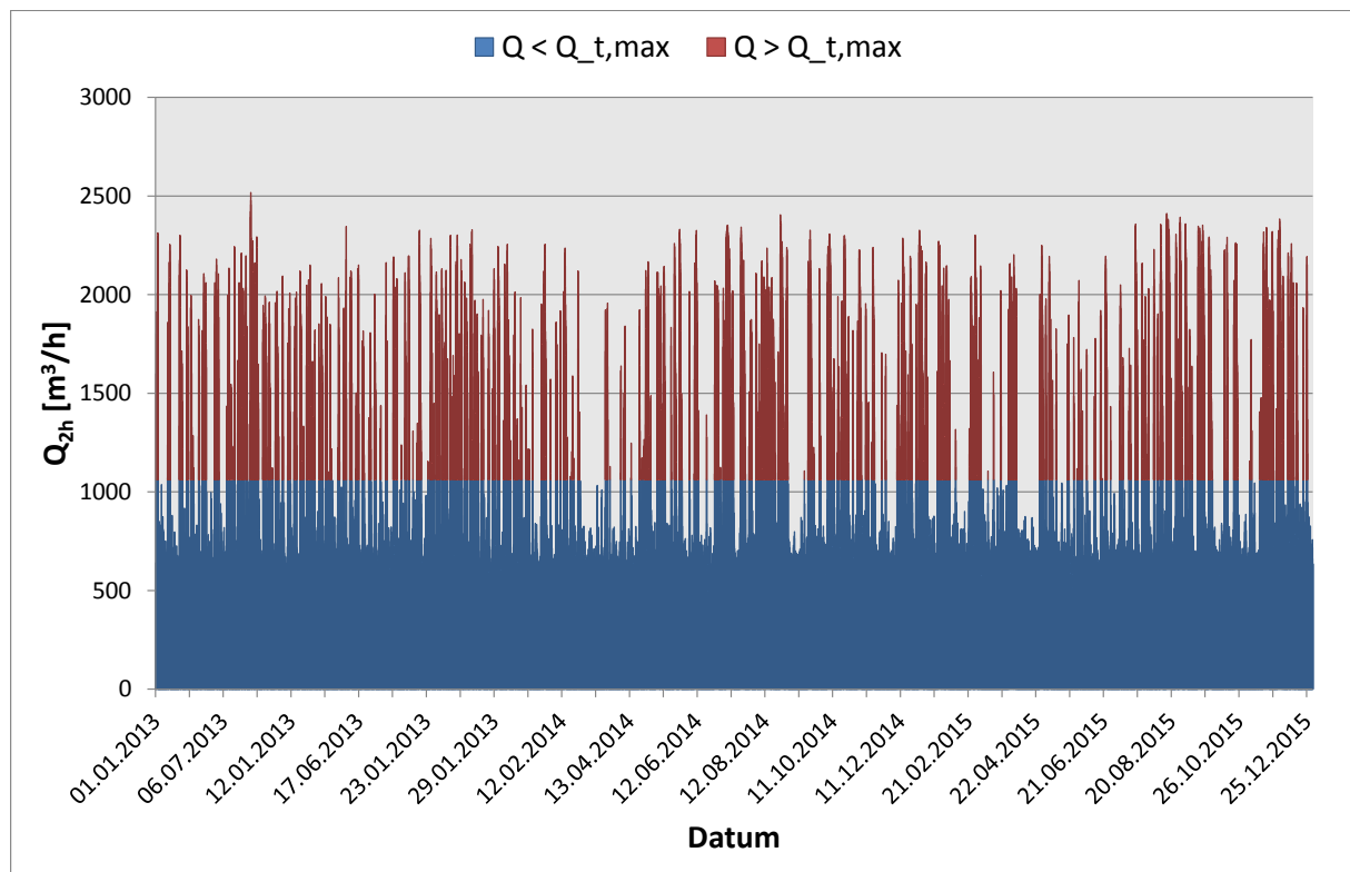
Abbildung 34: gemessene Zulaufmengen des GWK Kenten mit bei Teilstrombehandlung behandeltem (blau) und nicht behandeltem Anteil (rot)
