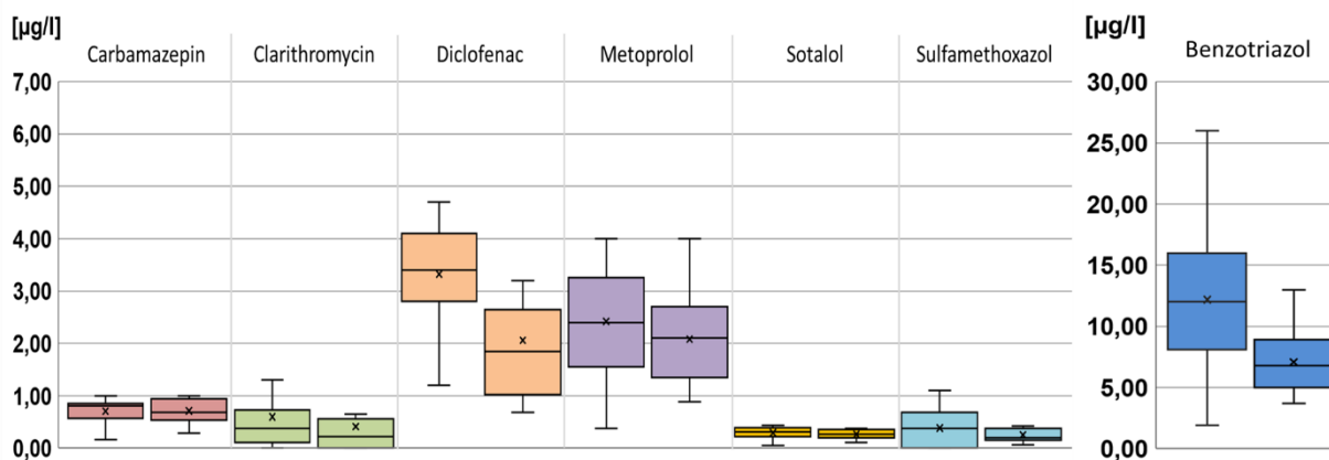
Abbildung 32: GWK Kenten, Zu- und Ablaufkonzentrationen der sieben Leitparameter
