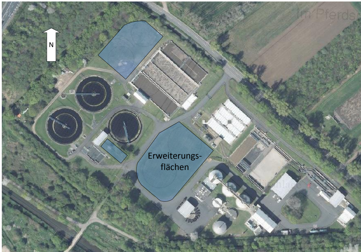
Abbildung 33: Erweiterungsflächen für die 4. Reinigungsstufe
