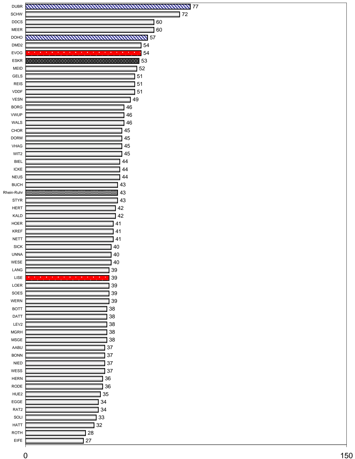
Abb. 3.6: Mittelwerte der Schwebstaubkonzentration in [µg/m³]; Rangfolge der Stationen im Messzeitraum April bis Juni 2000
