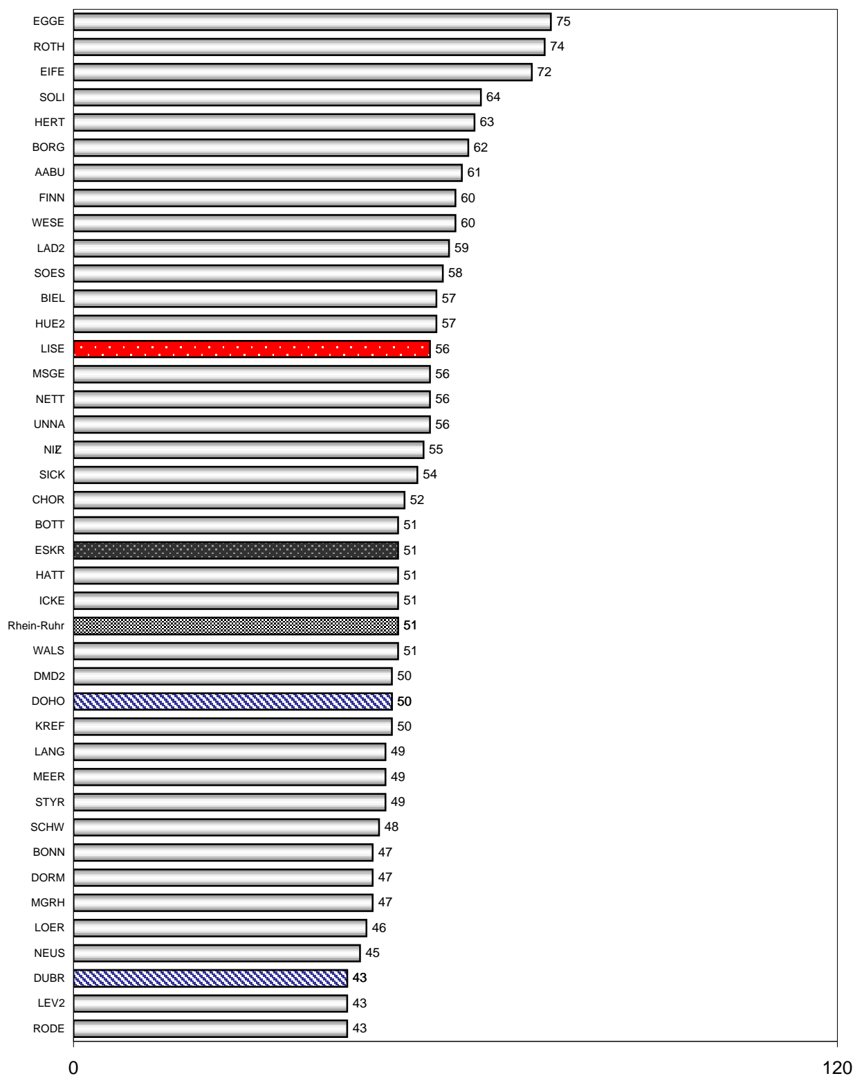
Abb. 3.5: Mittelwerte der Ozonkonzentration in [µg/m³]; Rangfolge der Stationen im Messzeitraum April bis Juni 2000
