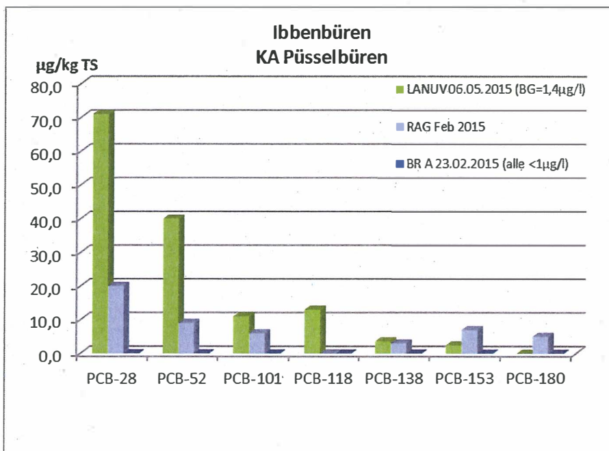
Abbildung 29: PCB-Konzentrationen im Grubenwasser des Oeynhaus-Stollen, Bergwerks-KA Püsselbüren
